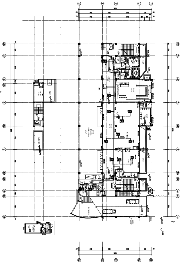
001-1 設備層樓梯及梯井平面圖
