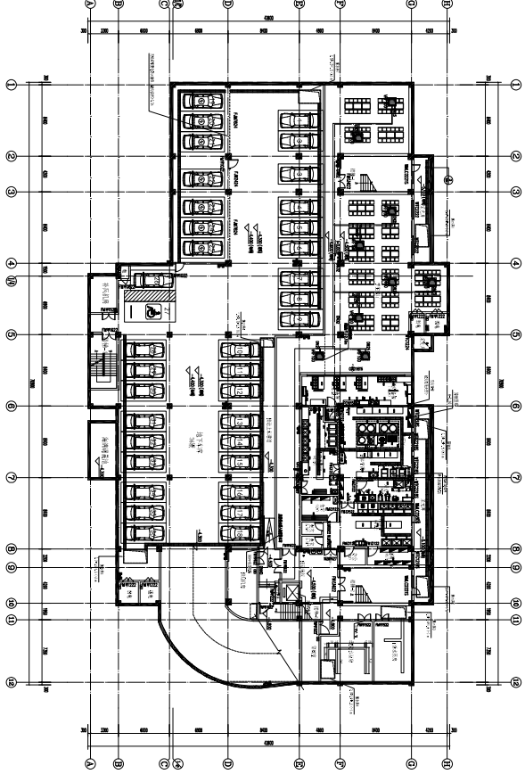
地下室各層設備層平面圖 1:150
