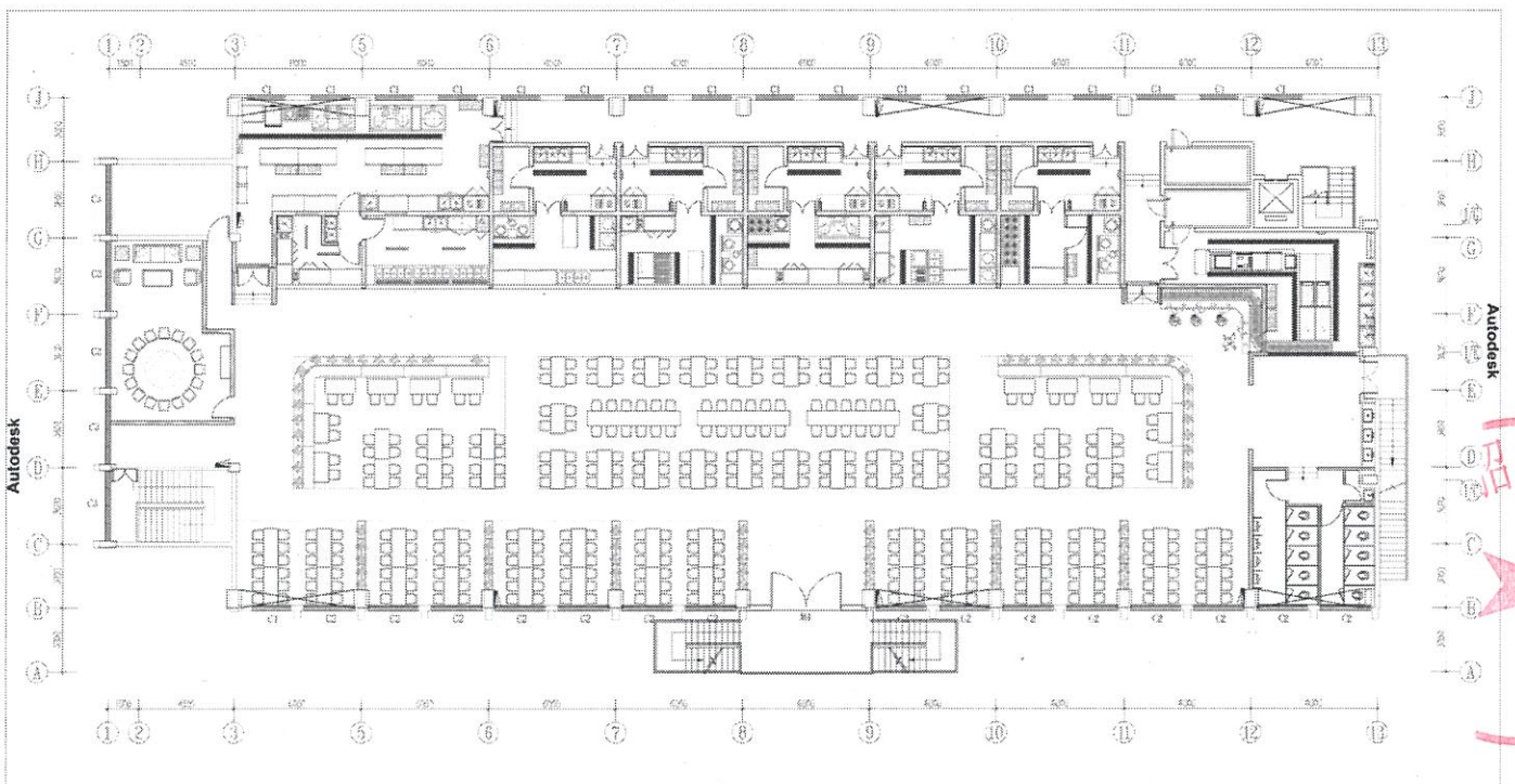
(2) 食堂二层图纸
