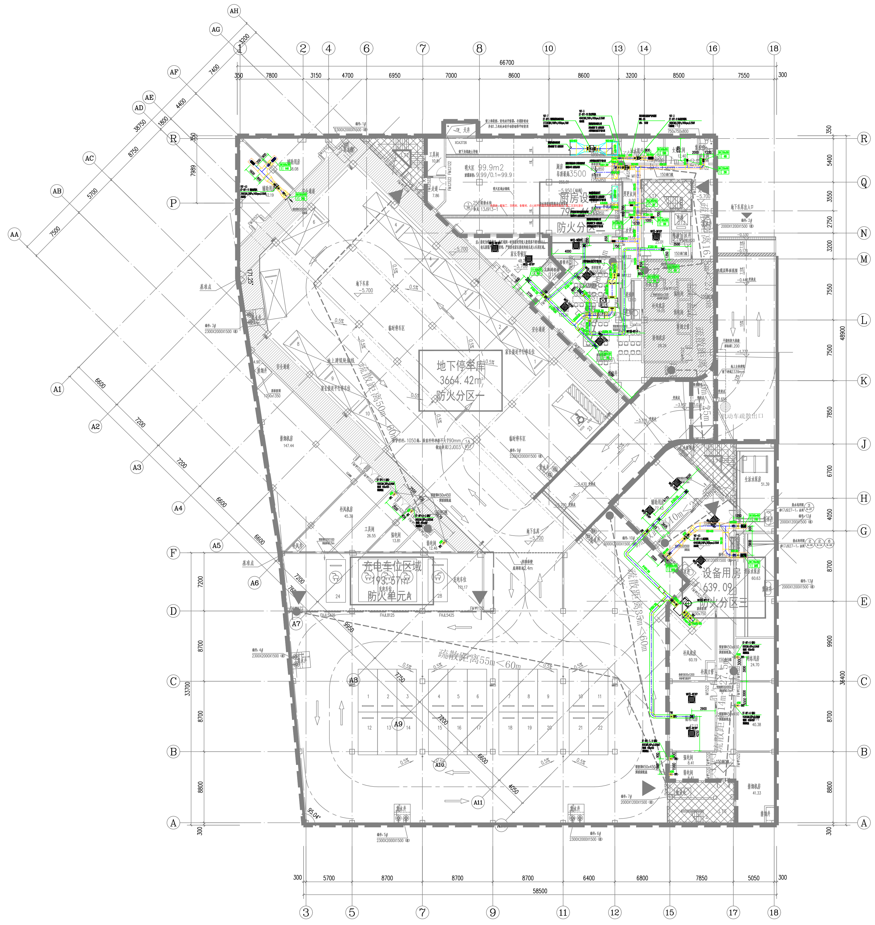
地下一层空调通风平面图 1:100
