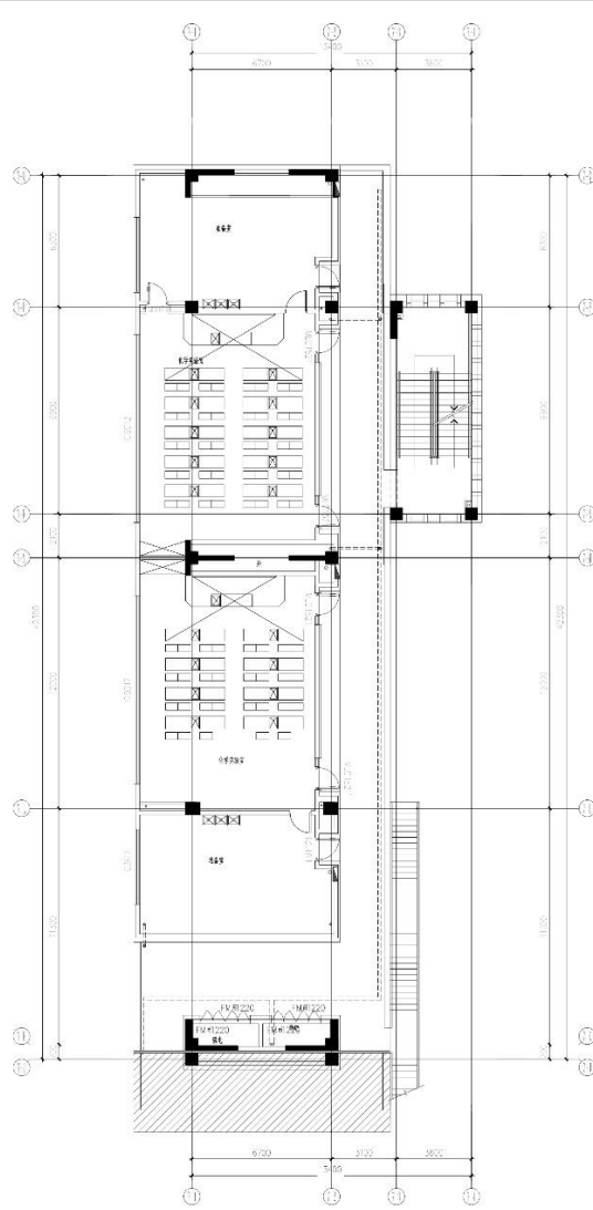
二层平面图 1:100
