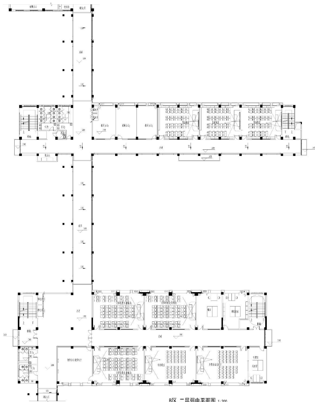
B区 二层弱电平面图 1:200
