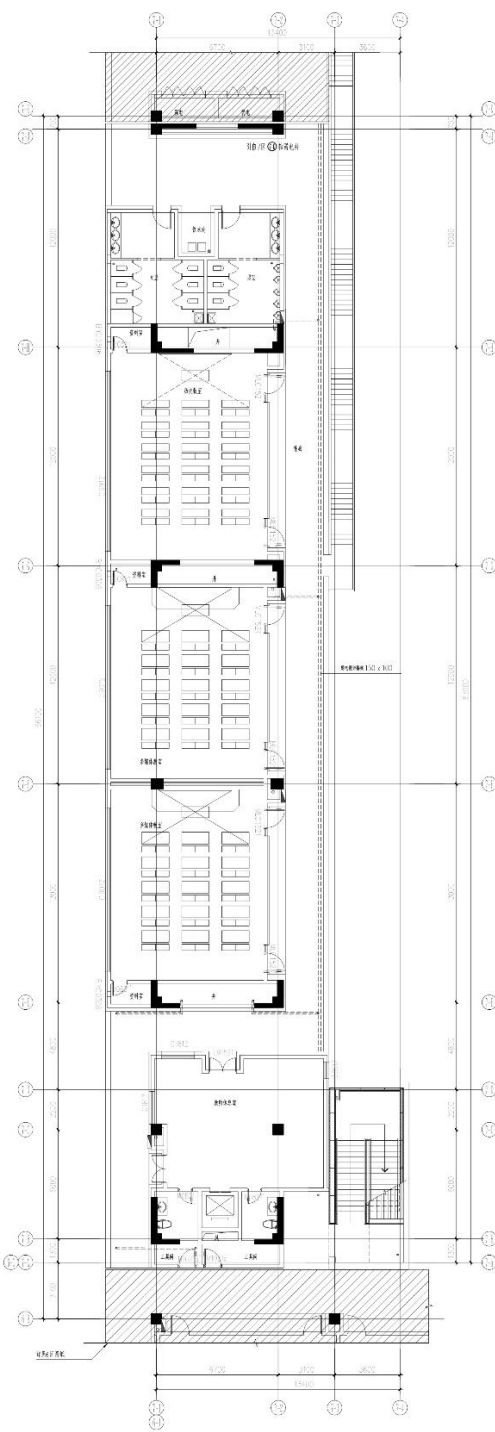
7F ②-③ 第二层标准e平面图 1:100
