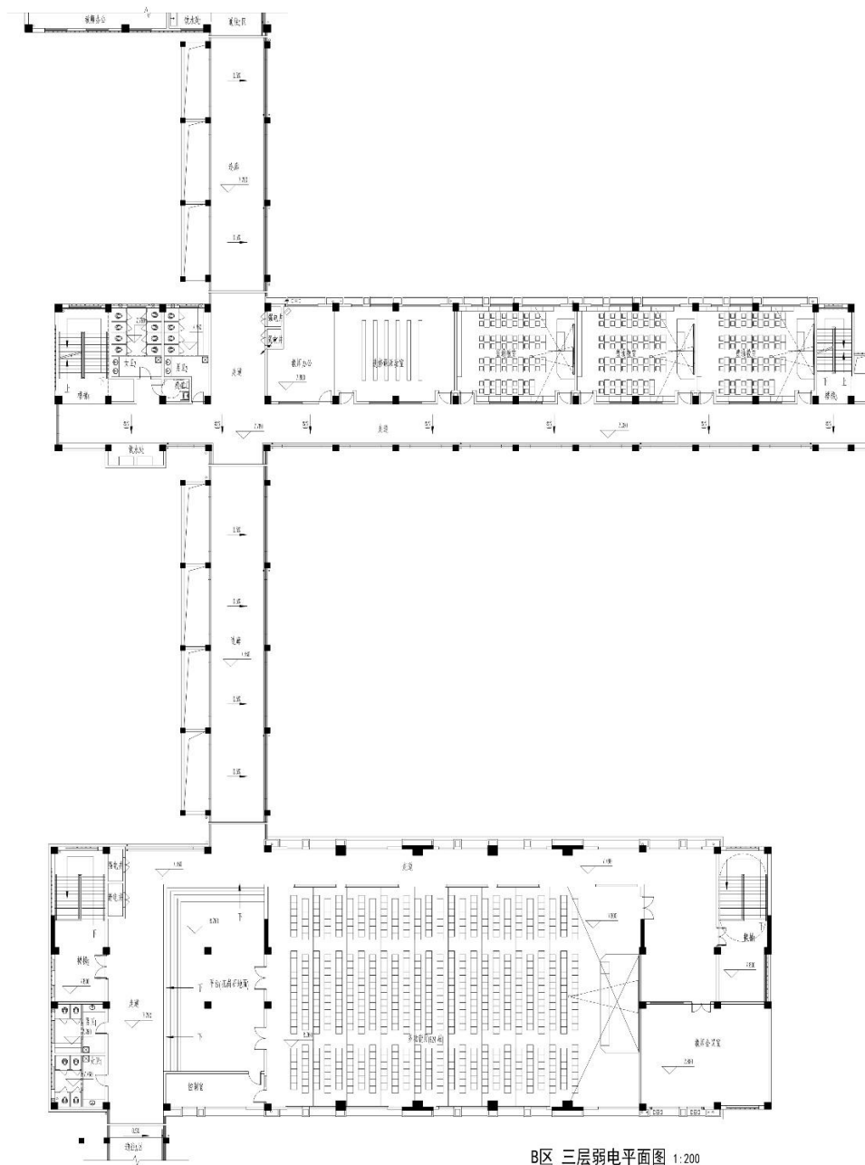
B区 三层弱电平面图 1:200
