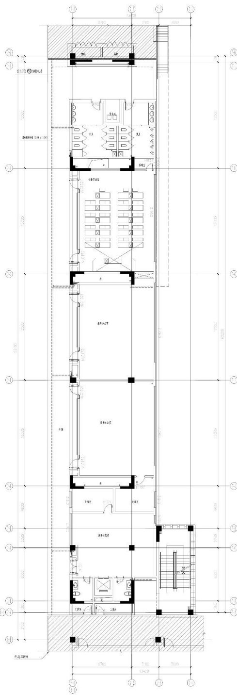
7F ②-② 楼二层弱电平面图 1:100
