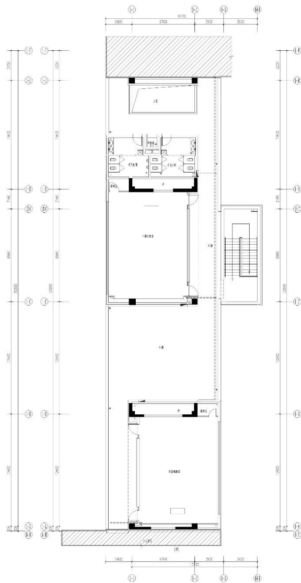
1E ⑪ 第二层教学平面图 1:100
