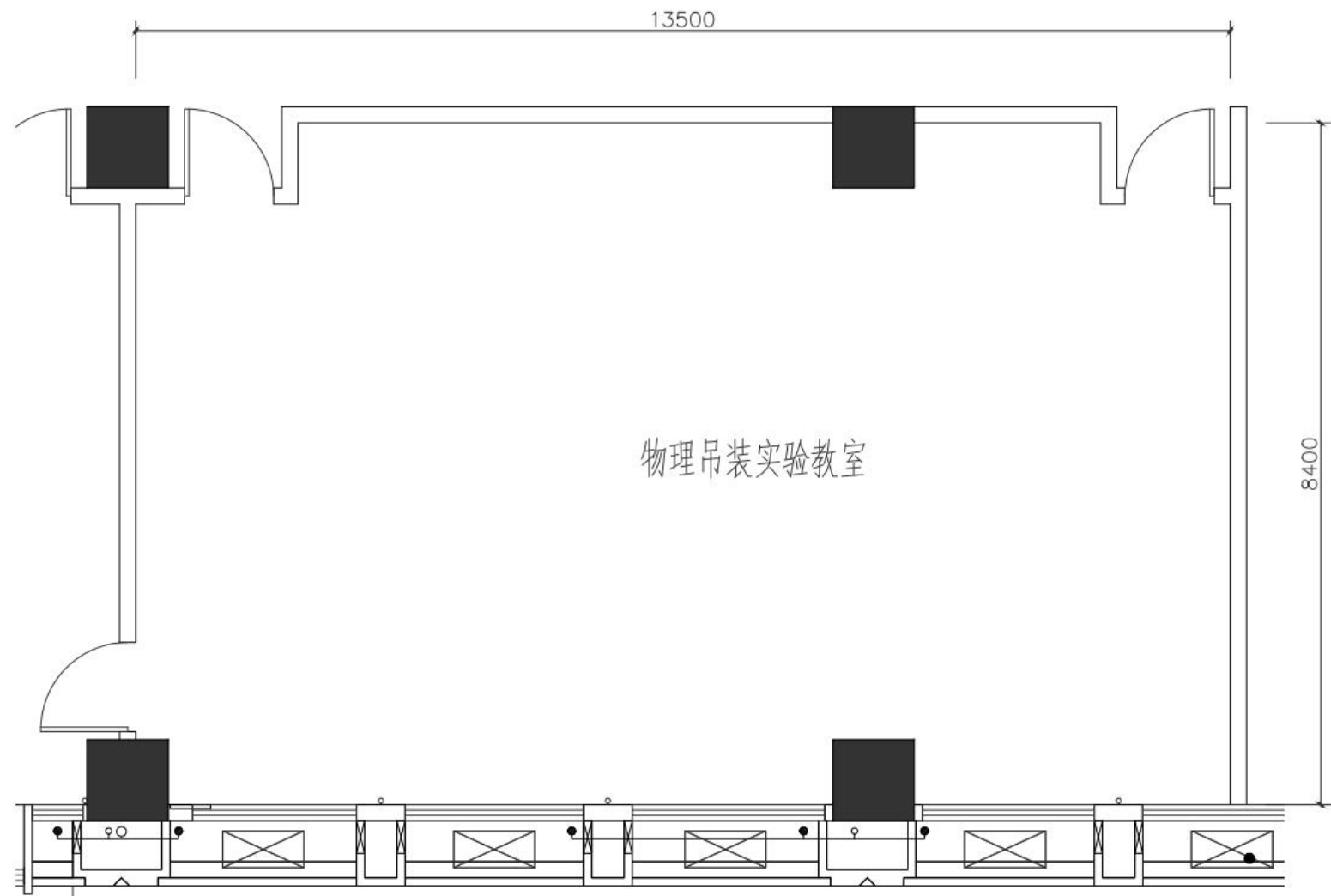
C 单元西片区规划学校“顶面供给物理实验室”平面框图
