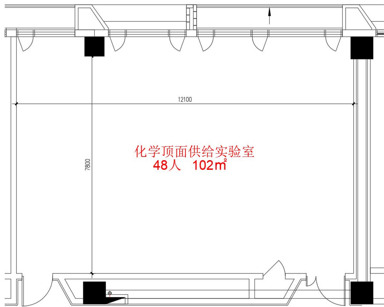
凌云路街道 419 街坊 3 丘地块学校“顶面供给化学实验室” 平面框图
