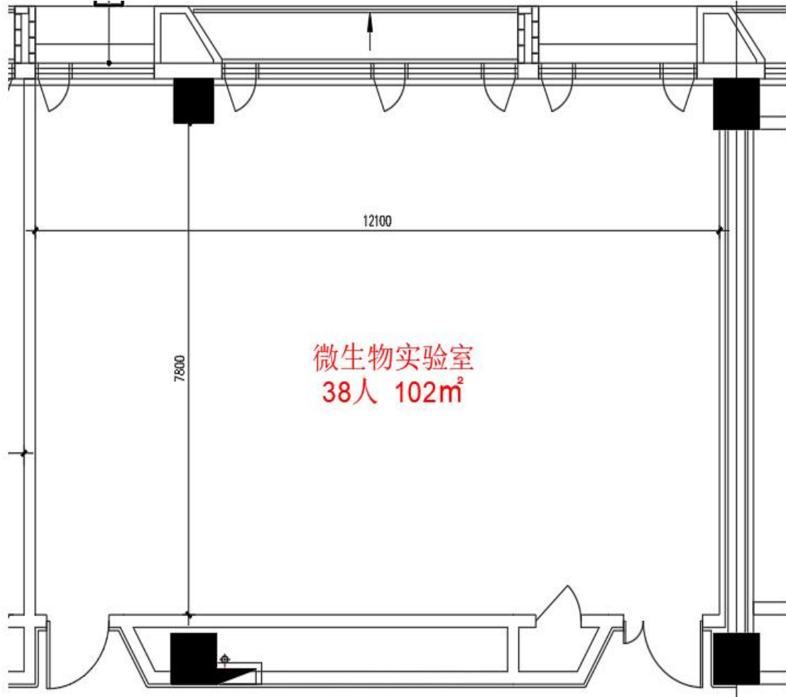
凌云路街道 419 街坊 3 丘地块学校“生物准备室”及“微生物实验室” 平面框图
