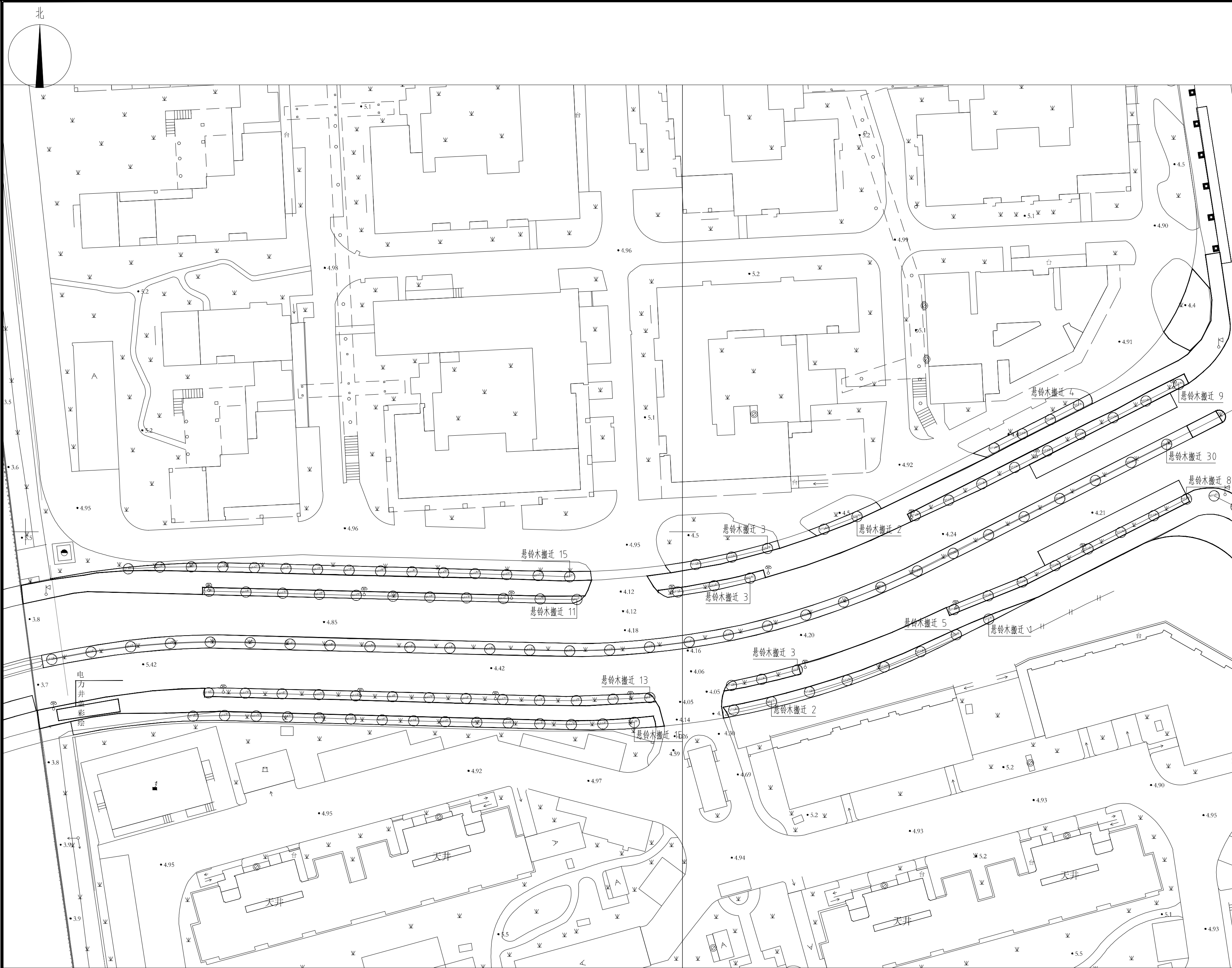
科农路（申江路-孙农路）绿化现状图（一） 1: 500
