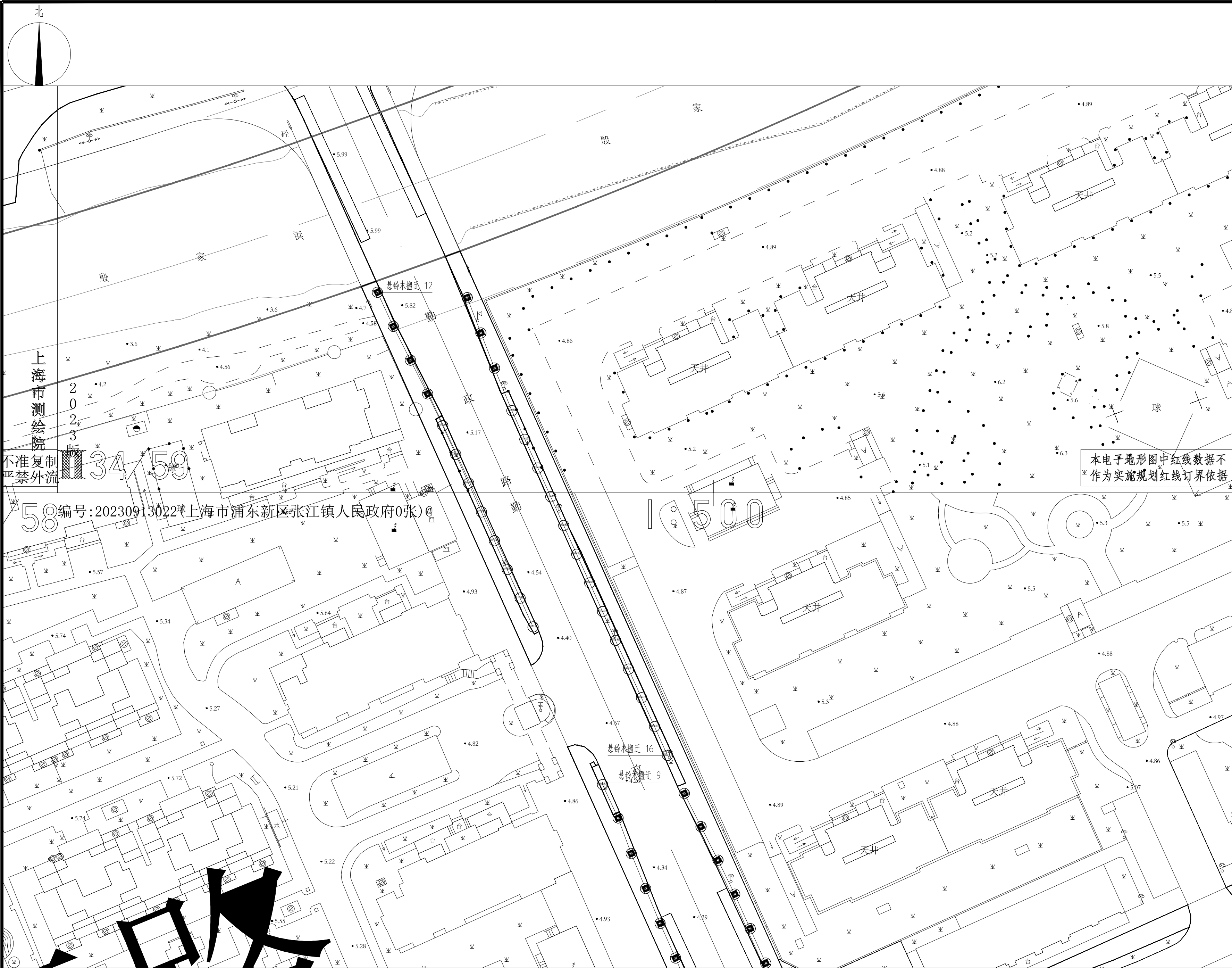
勤政路（军民公路—科农路）绿化现状图（一） 1：500
