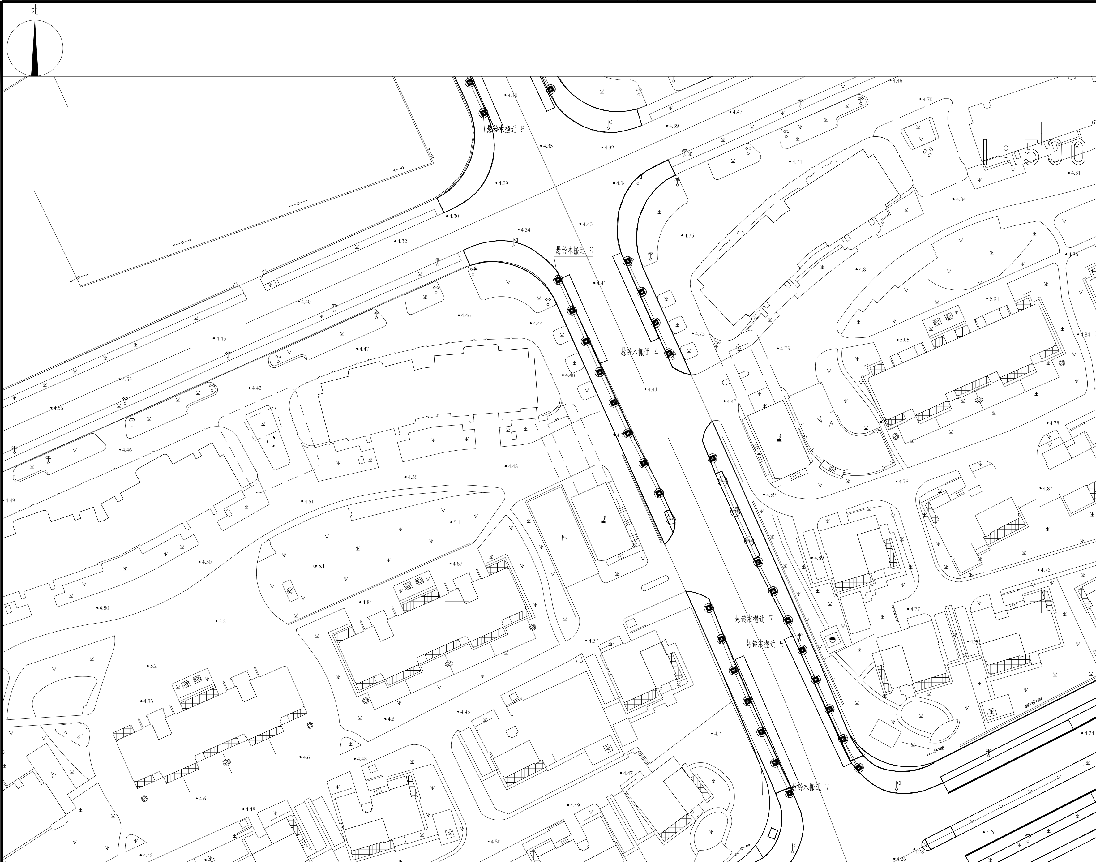
勤政路（军民公路—科农路）绿化现状图（四） 1：500
