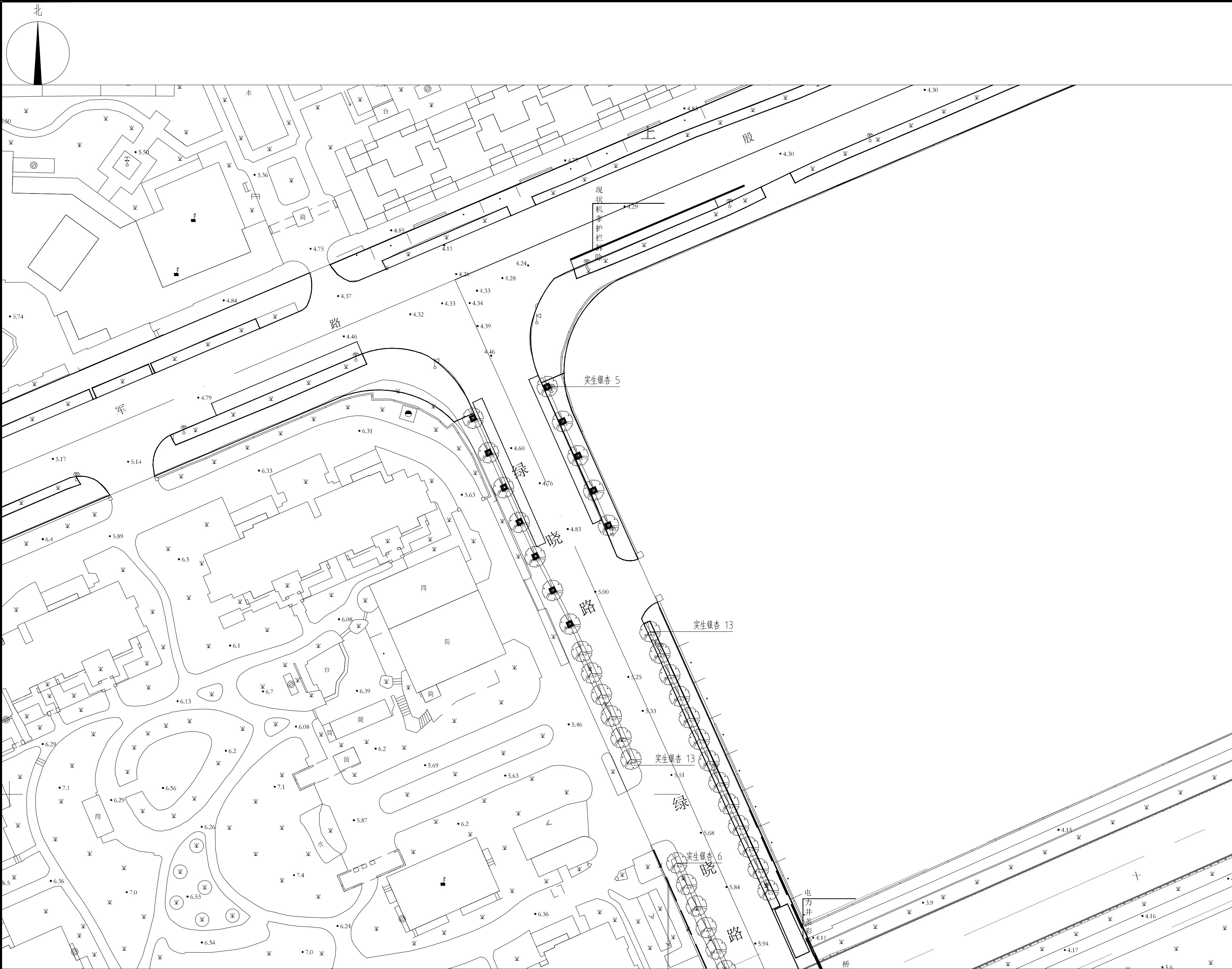
绿晓路（茂春路—科农路）绿化设计图（一） 1: 500
