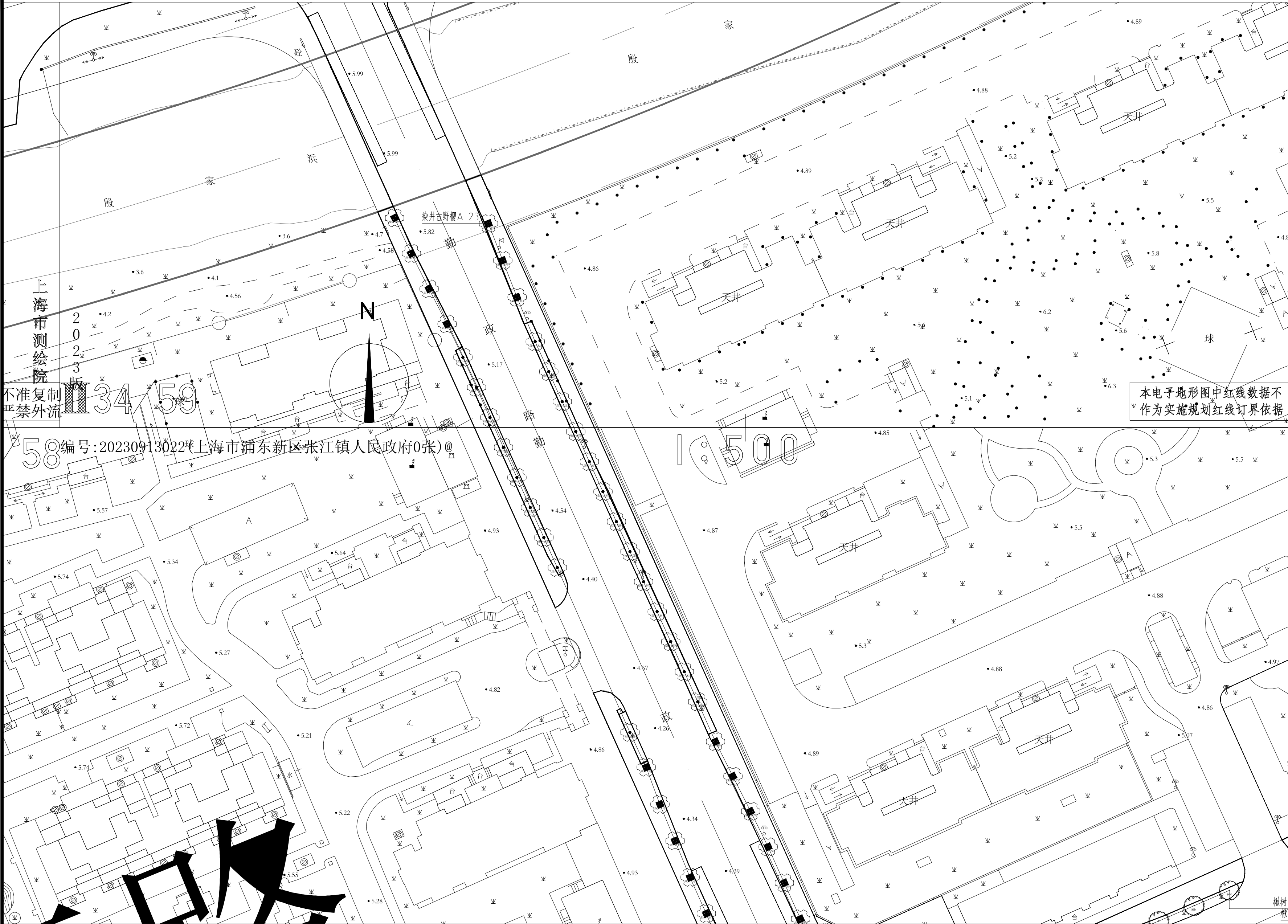
勤政路（军民公路—科农路）绿化设计图（一） 1：500
