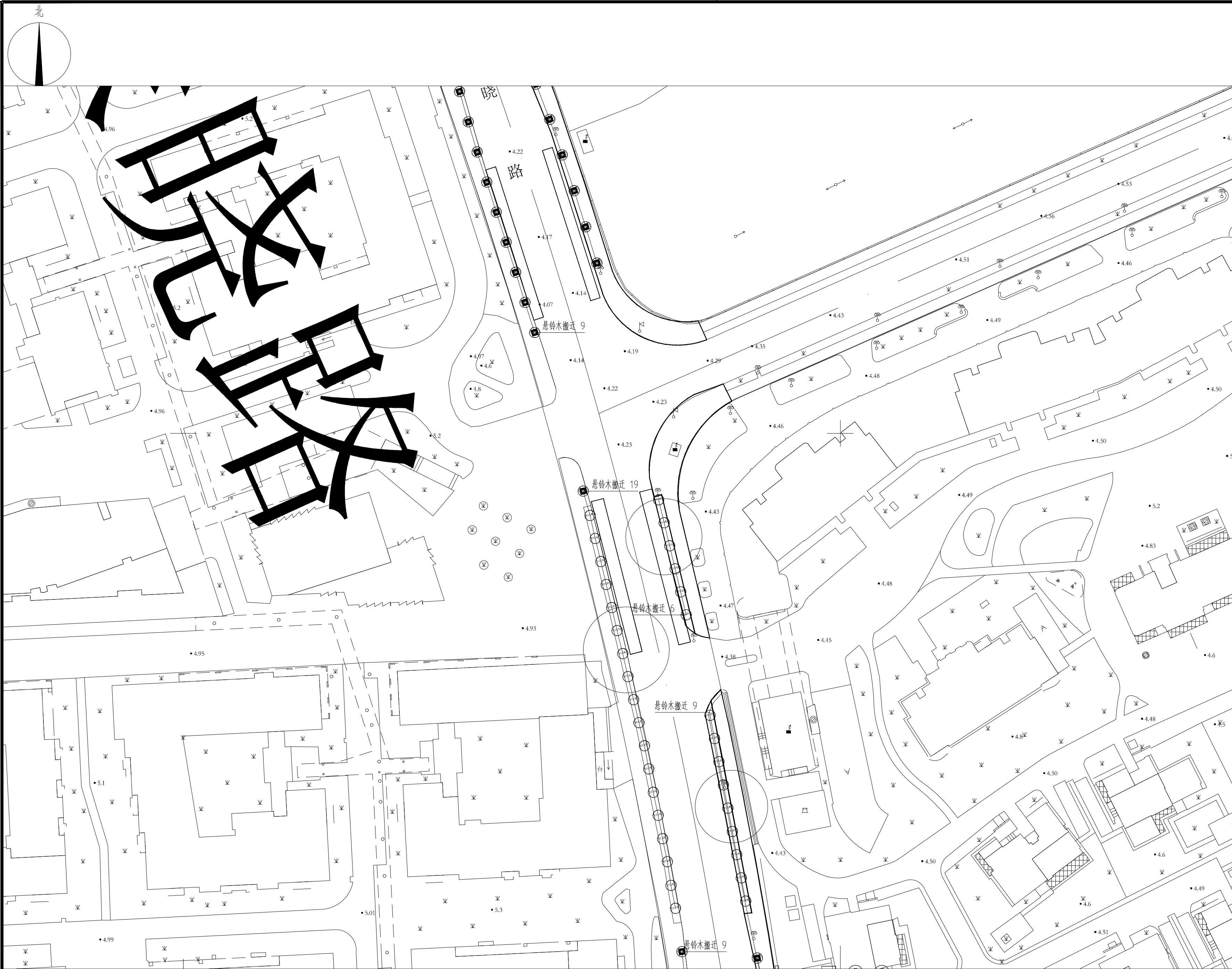
绿晓路（茂春路—科农路）绿化现状图（三） 1: 500
