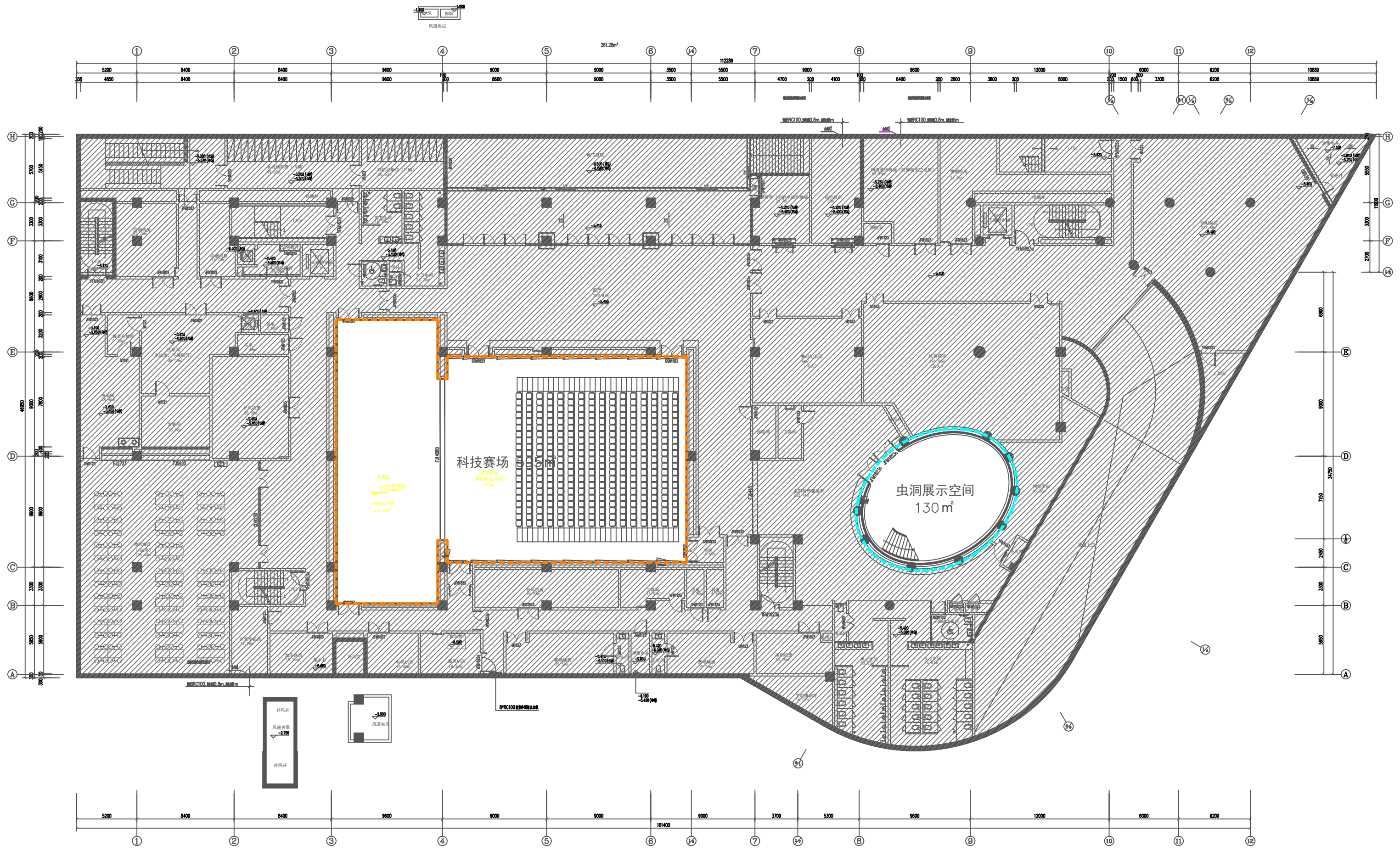
地下一层平面图
