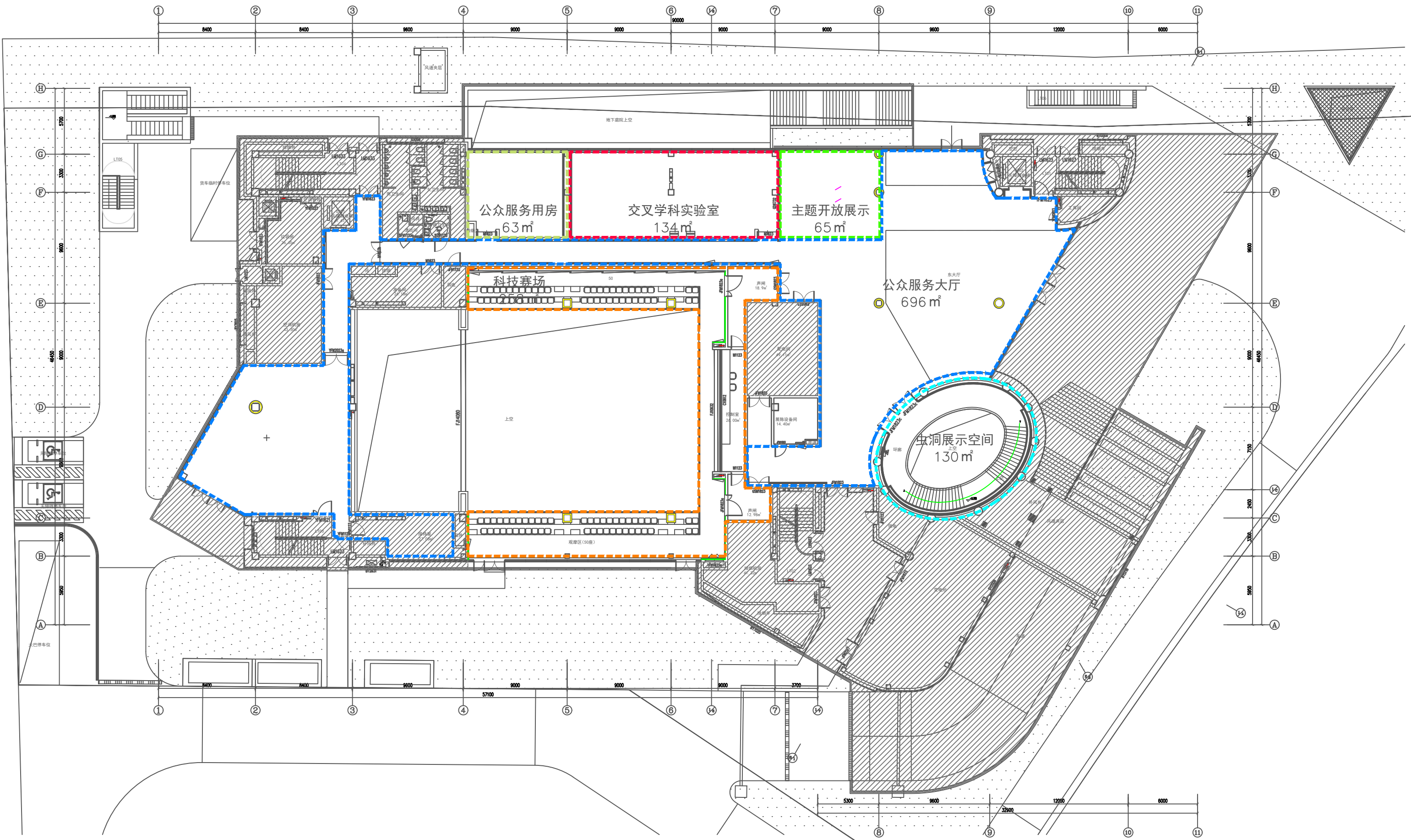
一层平面图
