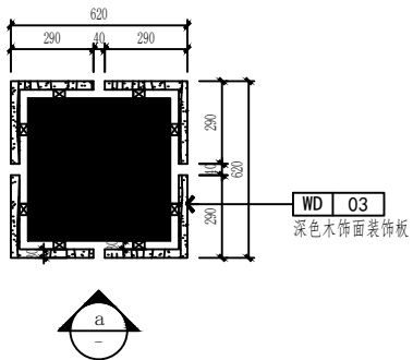
1 一层一门式大厅服务台平面图 1 P-11 LAYOUT PLAN SCALE 1:20
