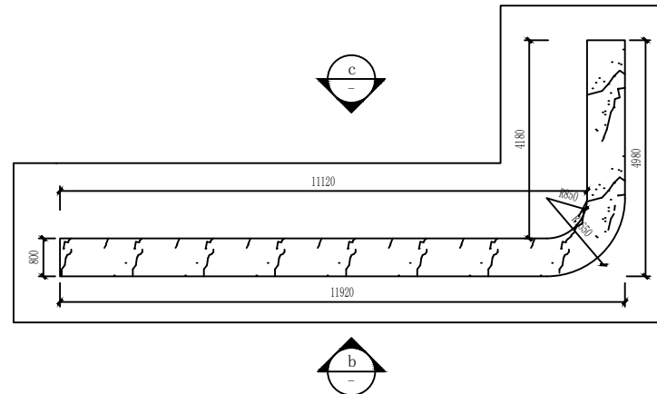
2 一层一门式大厅服务台平面图 2 P-11 LAYOUT PLAN SCALE 1:100
