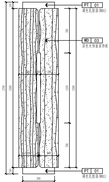
a 一层一门式大厅服务台立面图 a LAYOUT PLAN SCALE 1:20
