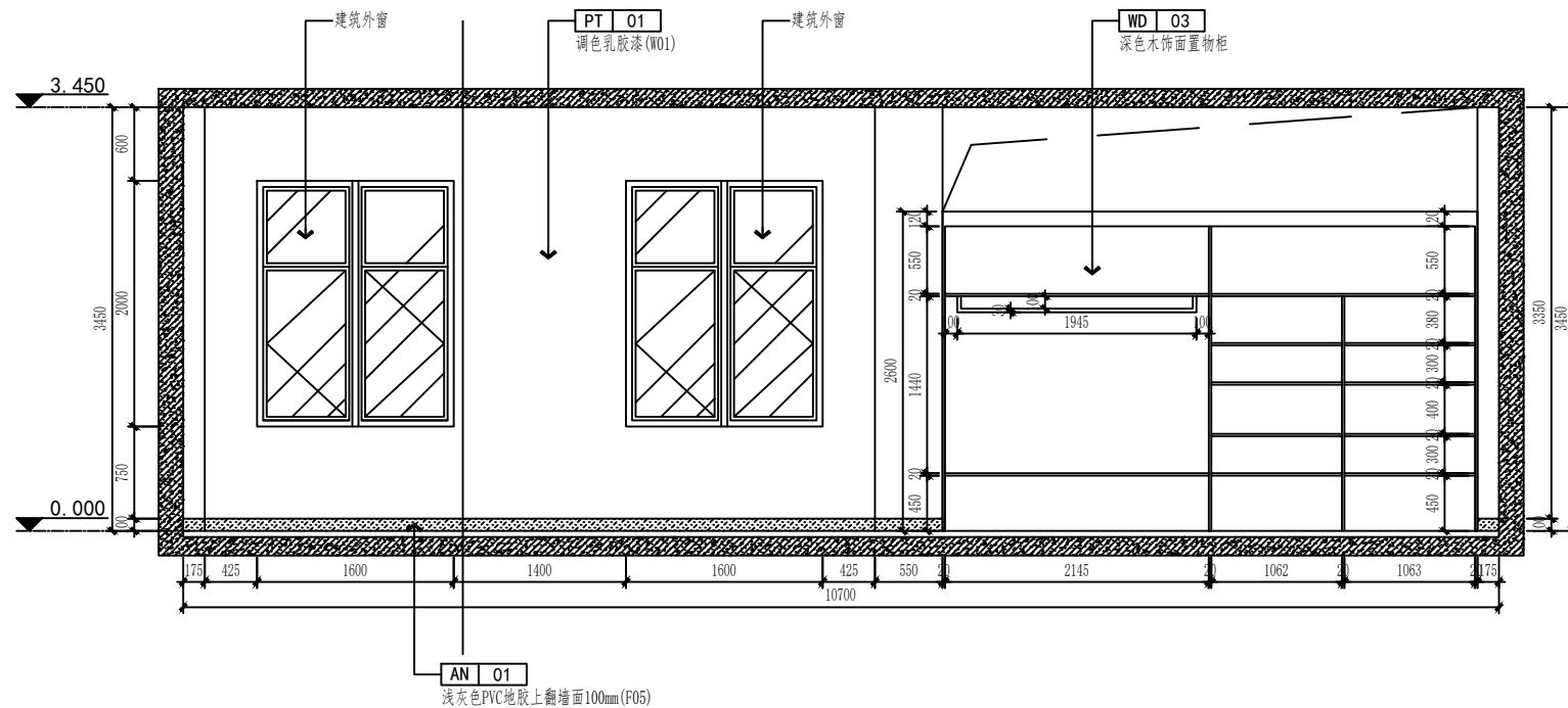
B 三层舞蹈室立面图 B P-33 LAYOUT PLAN SCALE 1:50
