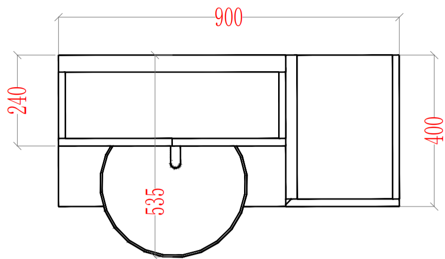
平面图
