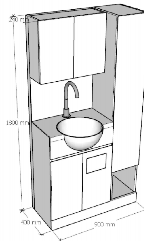
立体图
