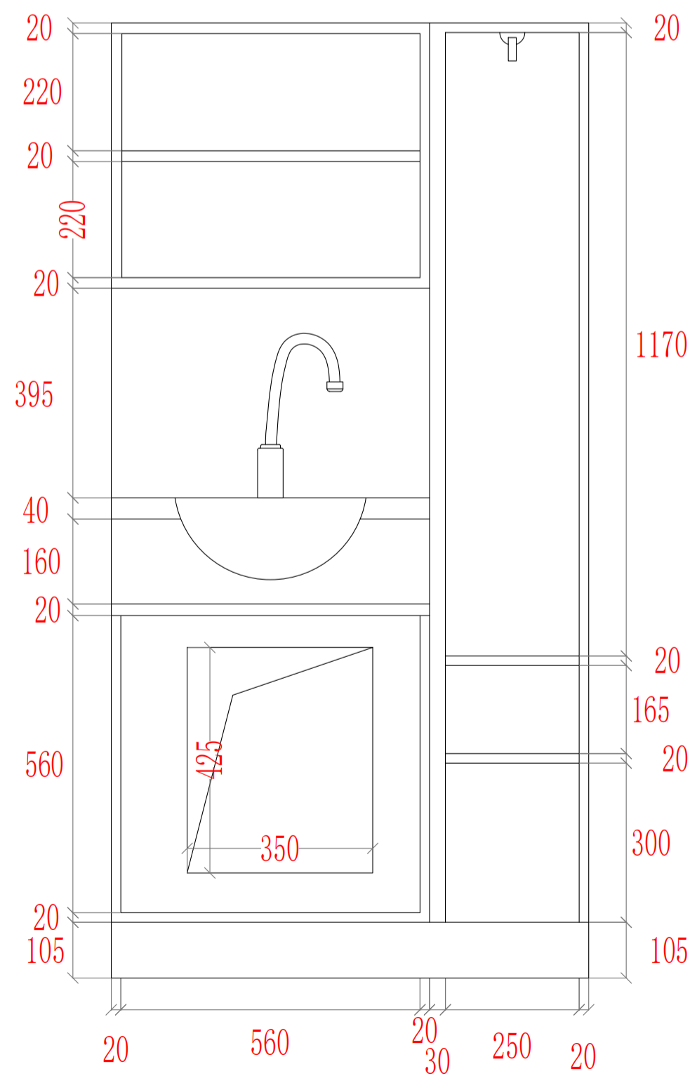
正视图
