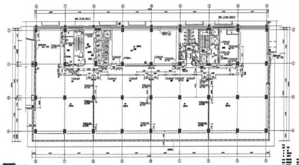
三层平面图
