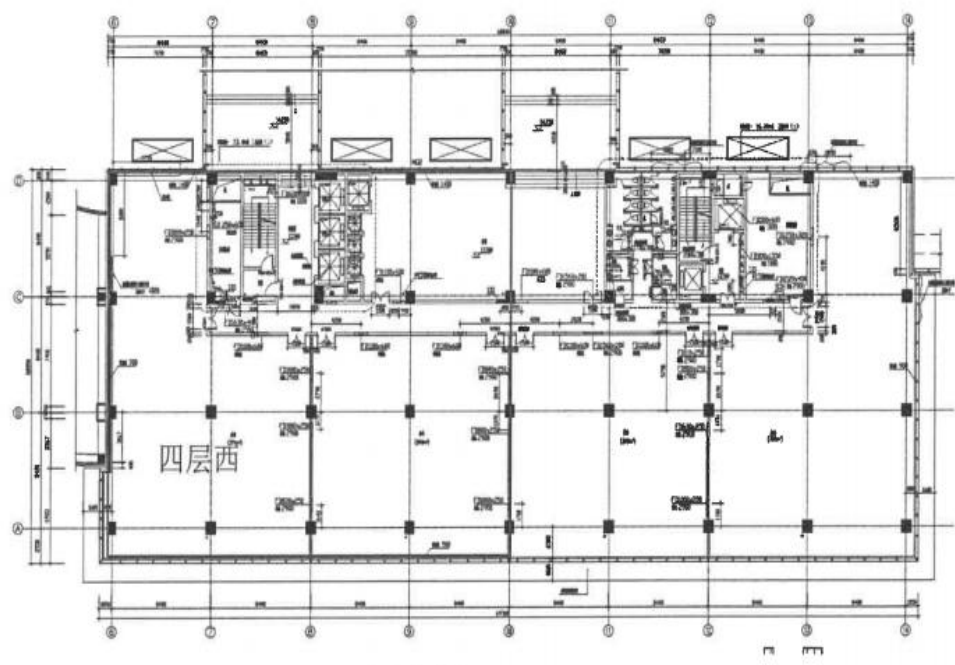
四层平面图
