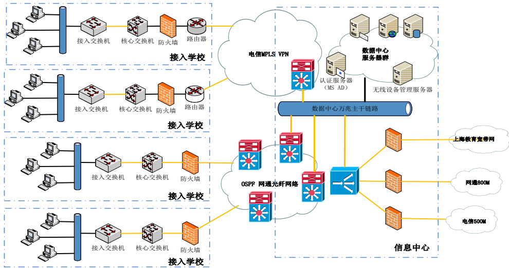
图 1 黄浦区教育城域网逻辑拓扑
