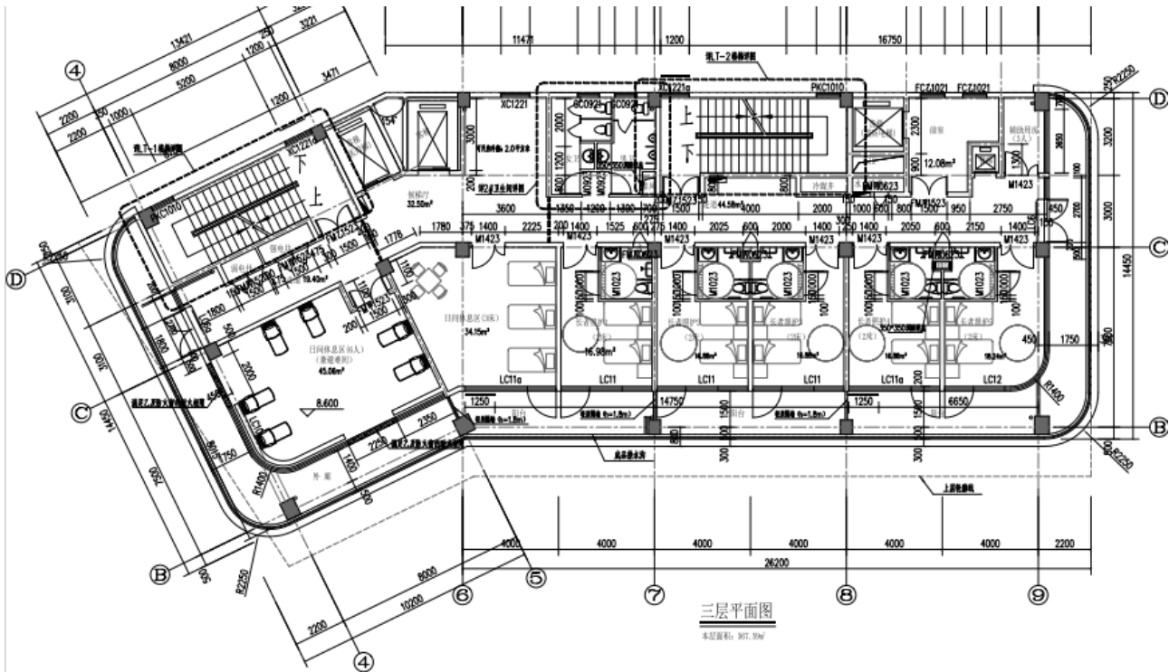
南区三层平面图
