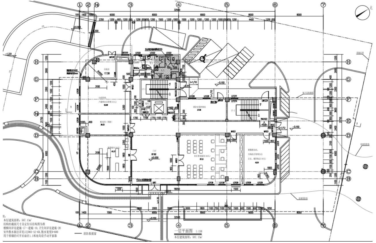
北区一层平面图
