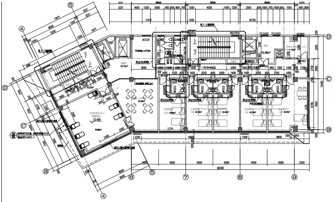
四层平面图
