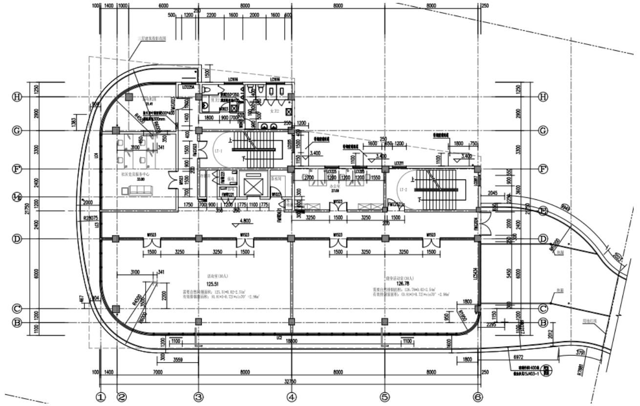
南区二层层平面图
