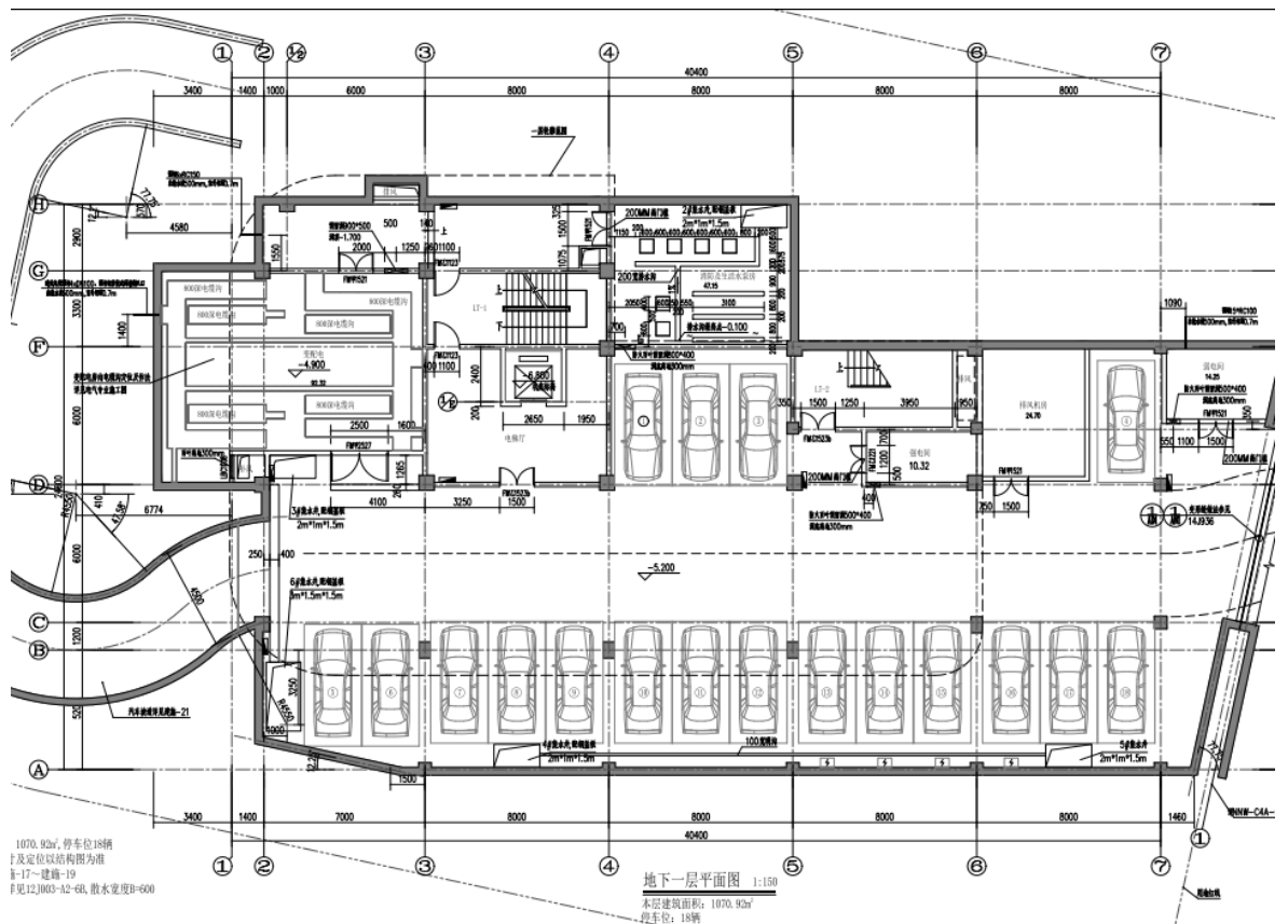
北楼地下一层层平面图
