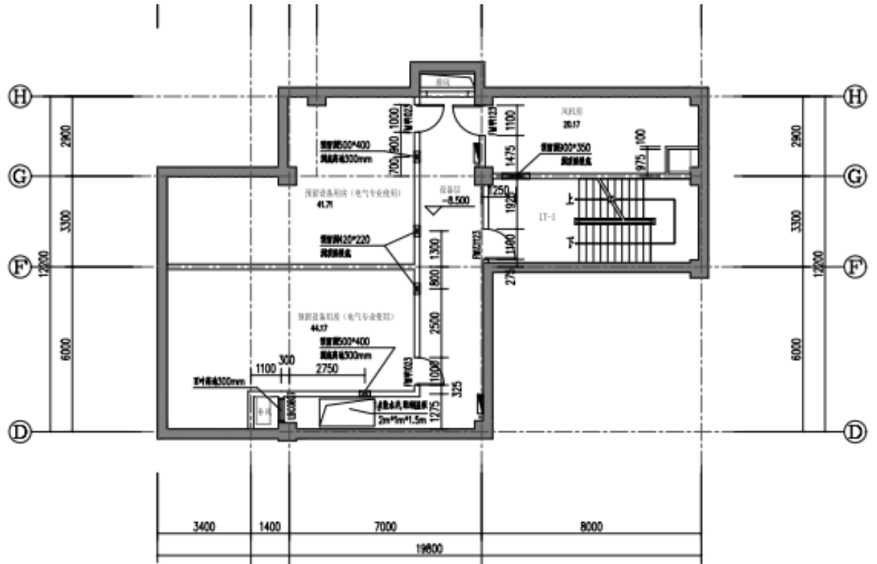
北楼地下二层平面图
