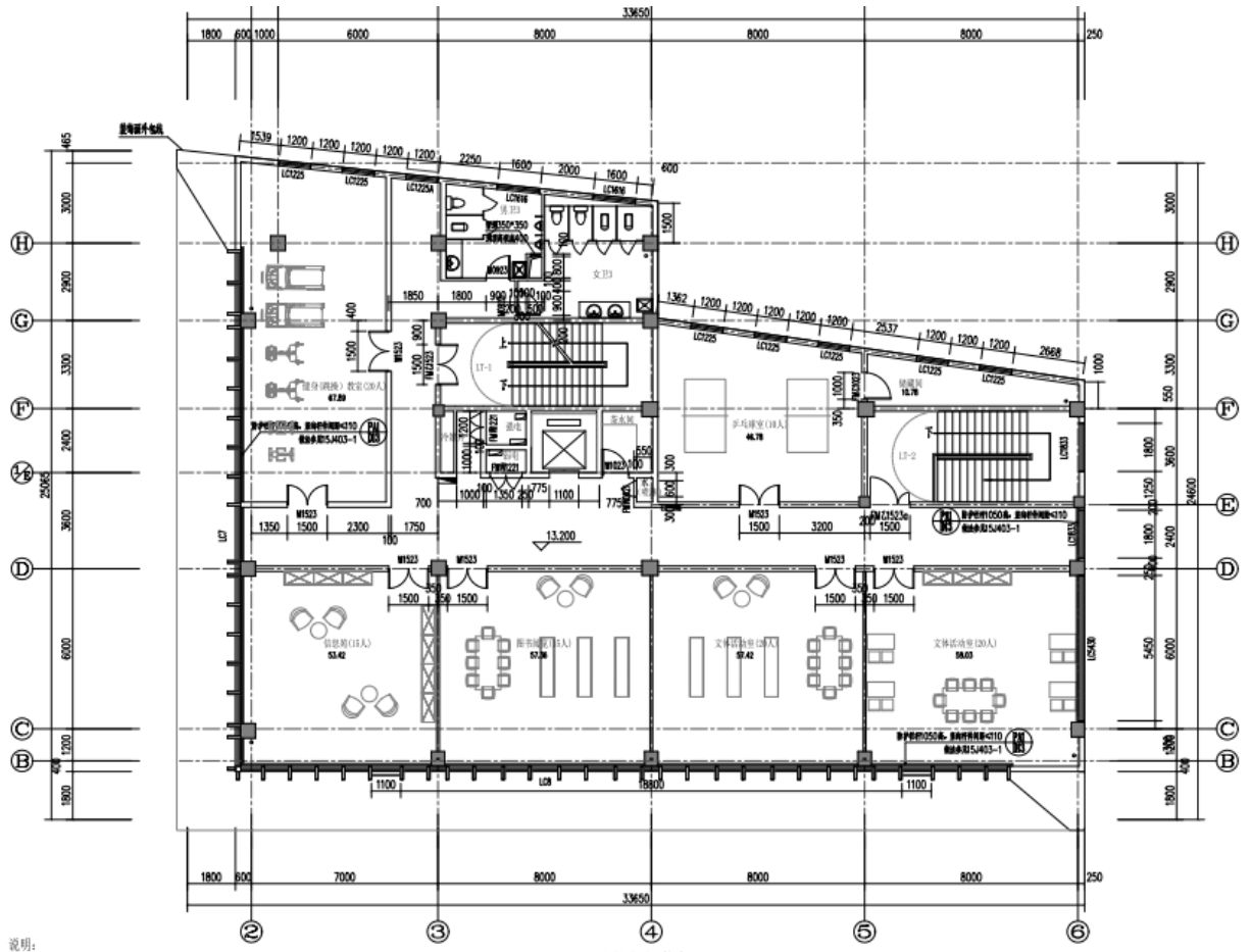
南区四层平面图
