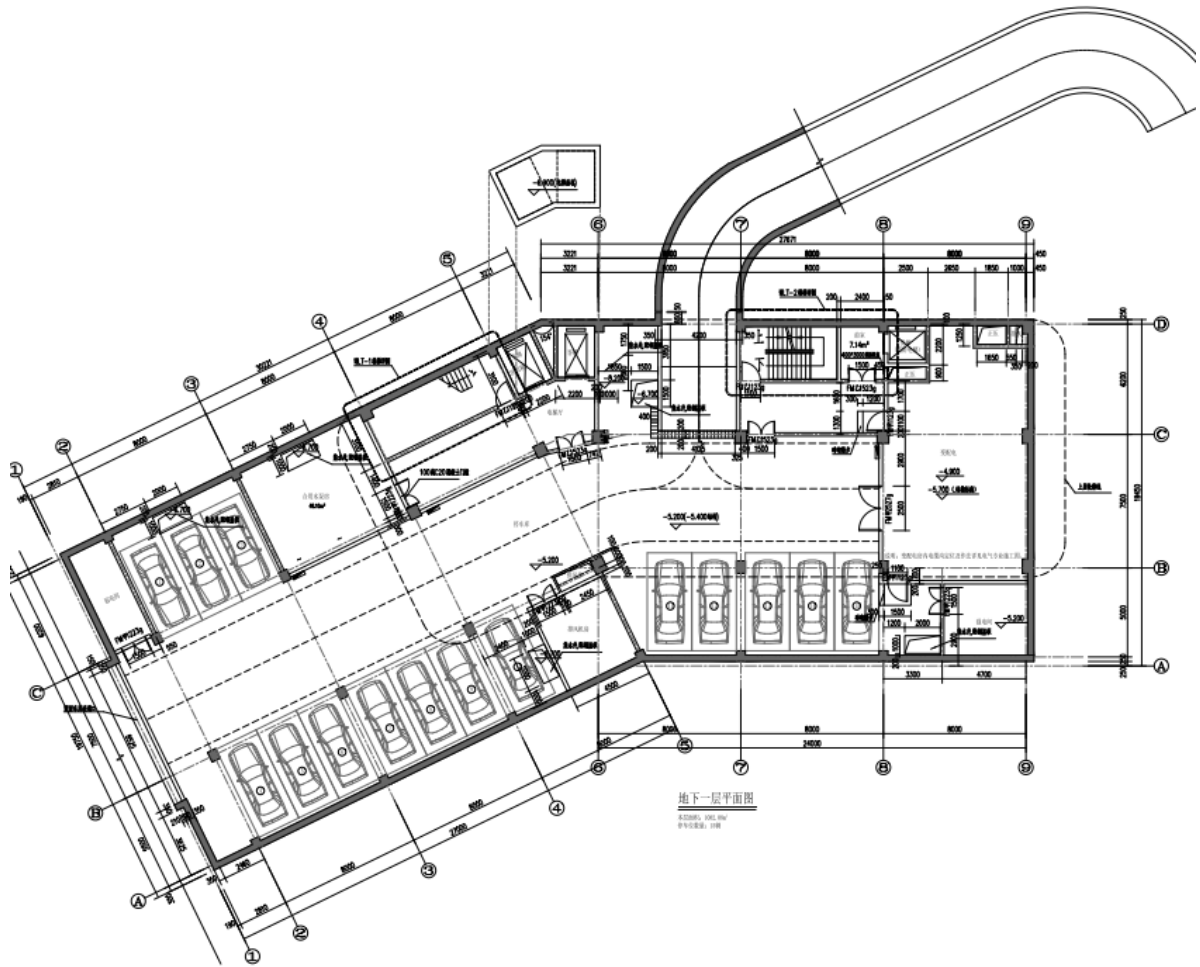
南区一层平面图
