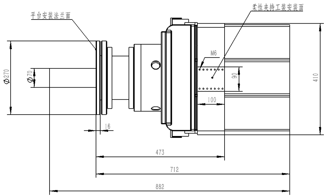
图 1 等离子体枪视图 1
