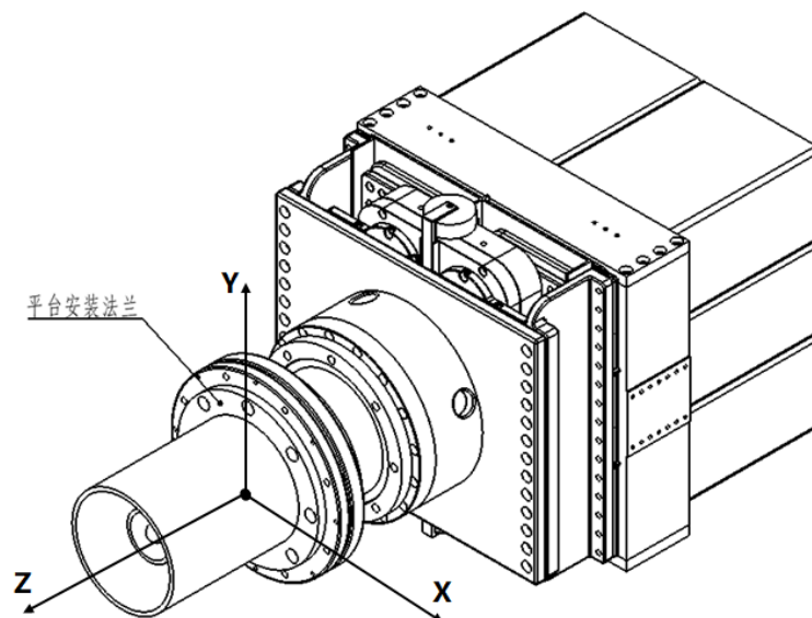
图3 等离子体枪与平台安装法兰连接示意图
