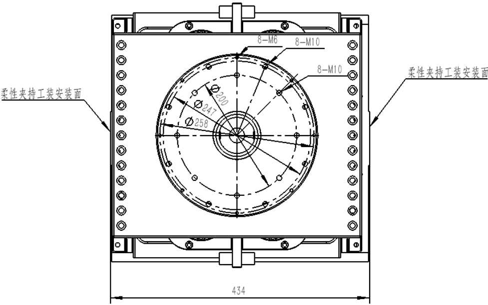
图 2 等离子体枪视图 2
