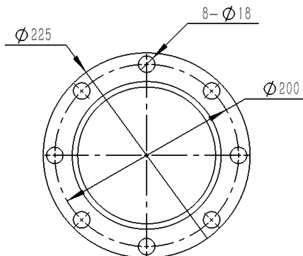
图4 平台安装法兰接口示意图
