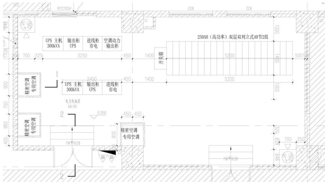
二号楼一层电力电池室平面图
