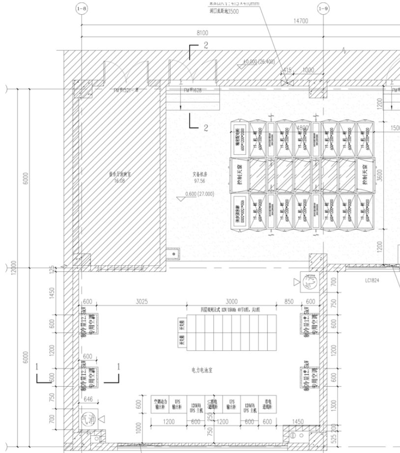
一号楼七层灾备机房及电力电池室平面图
