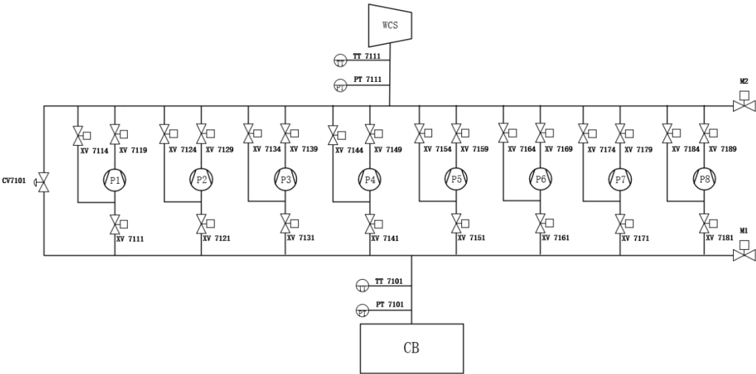
图 1 减压降温泵系统流程示意图
