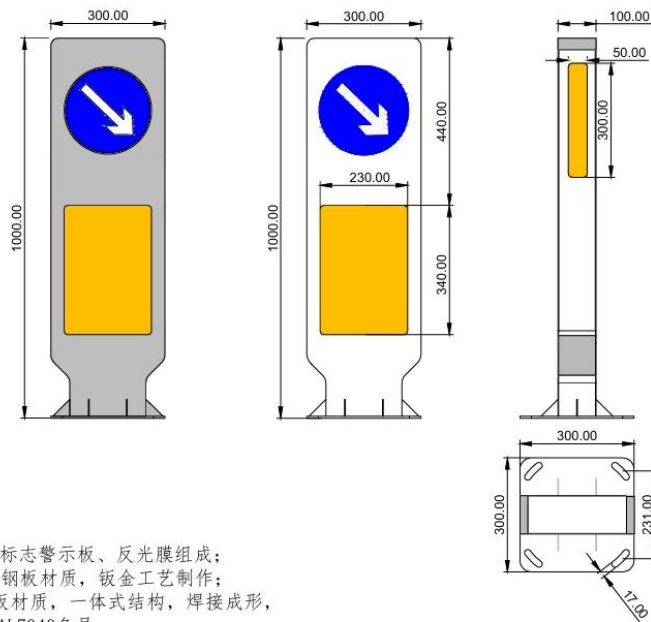
护栏反光端头（刚性）
