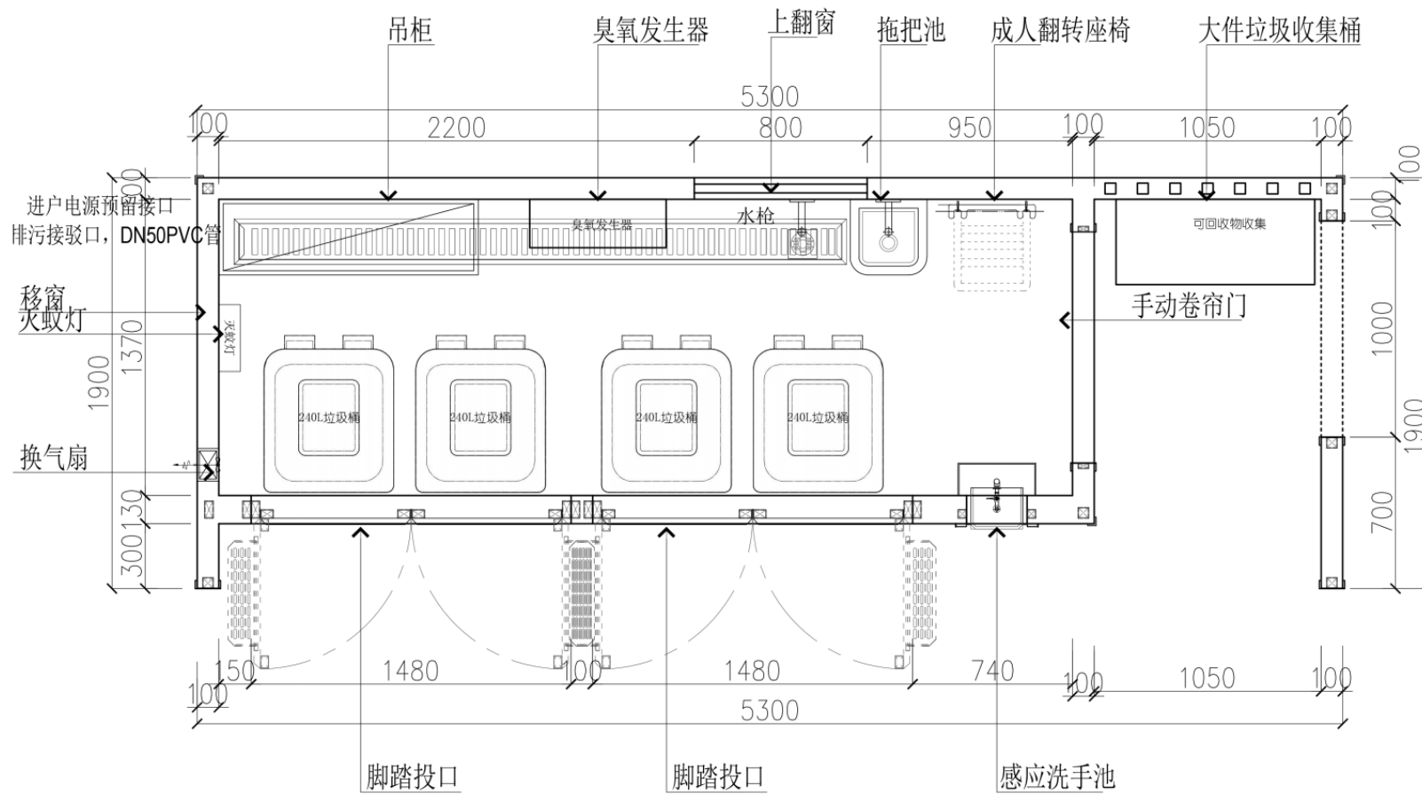
平面布置图
