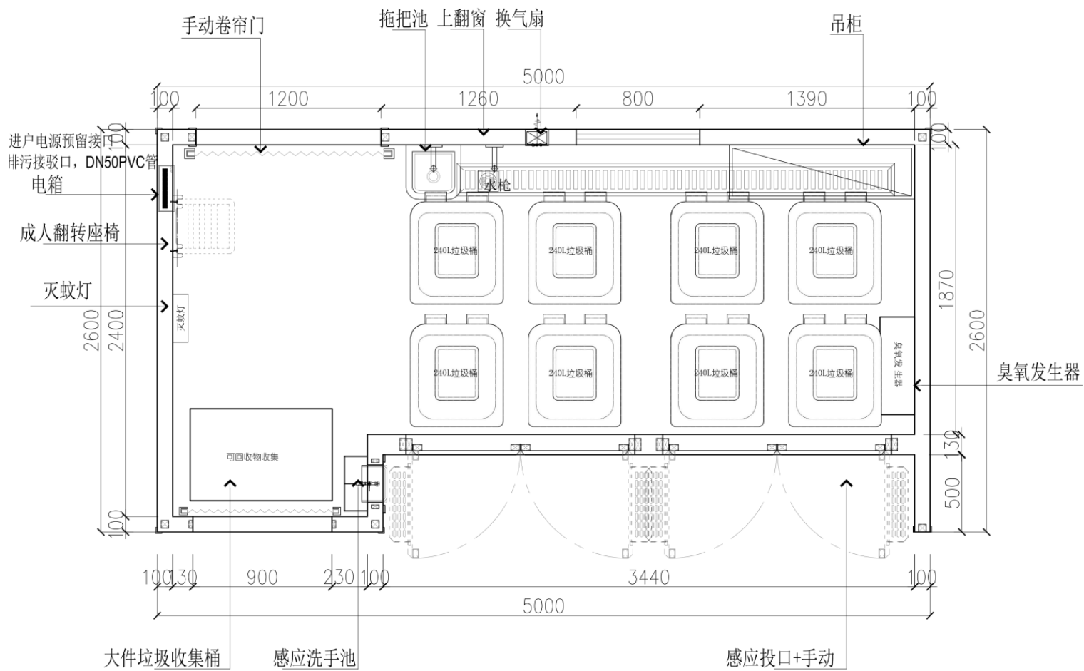
平面布置图
