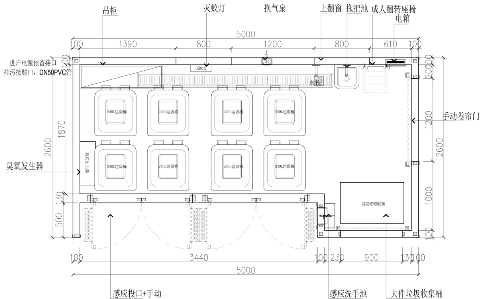
平面布置图
