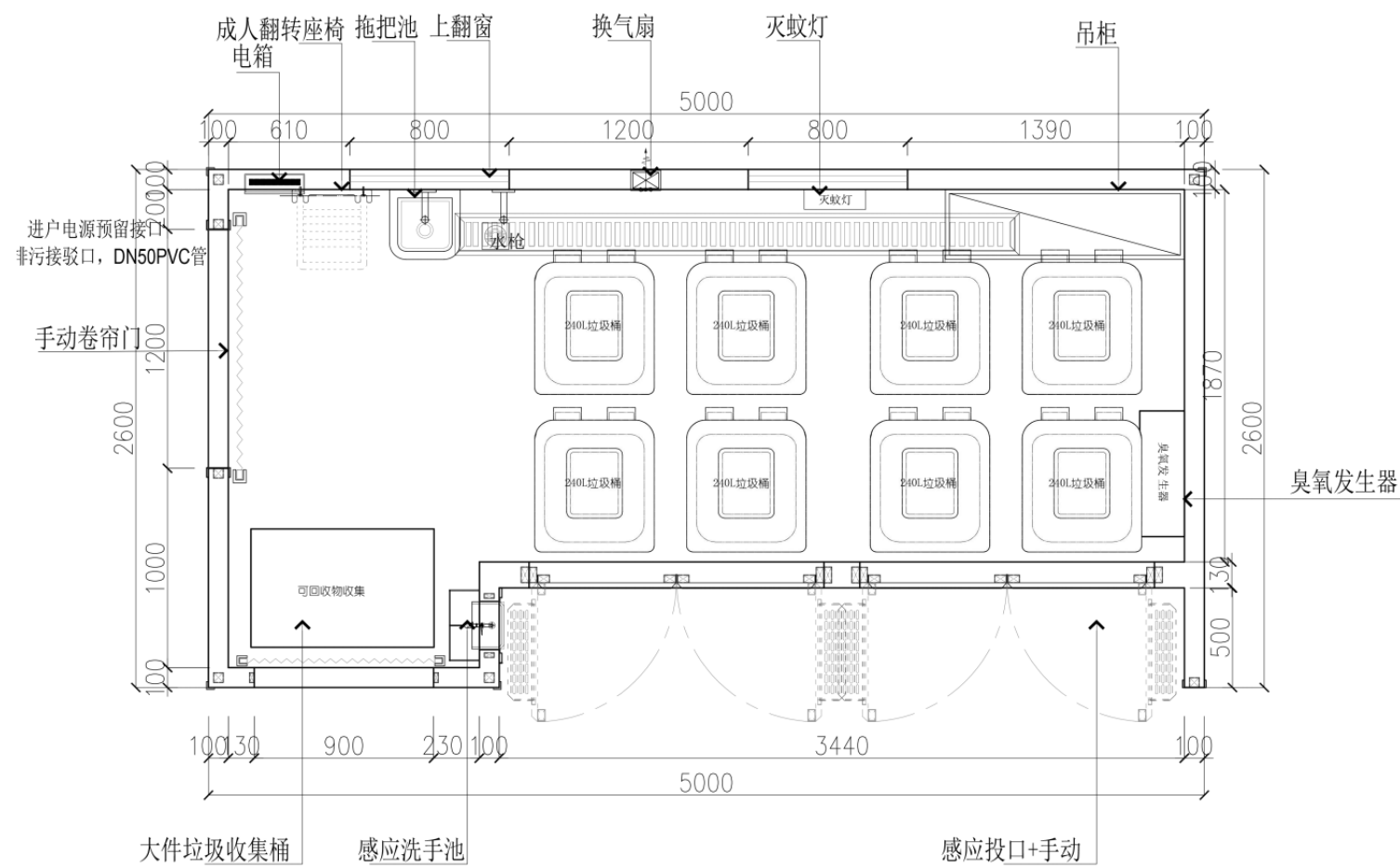
平面布置图
