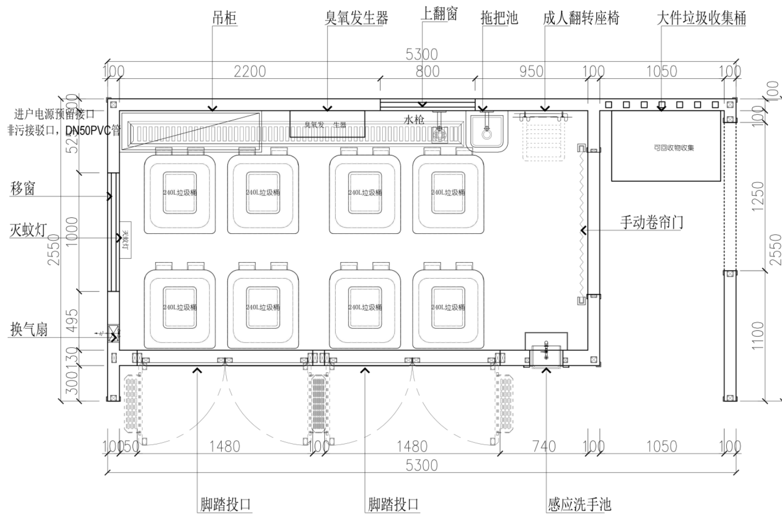
平面布置图
