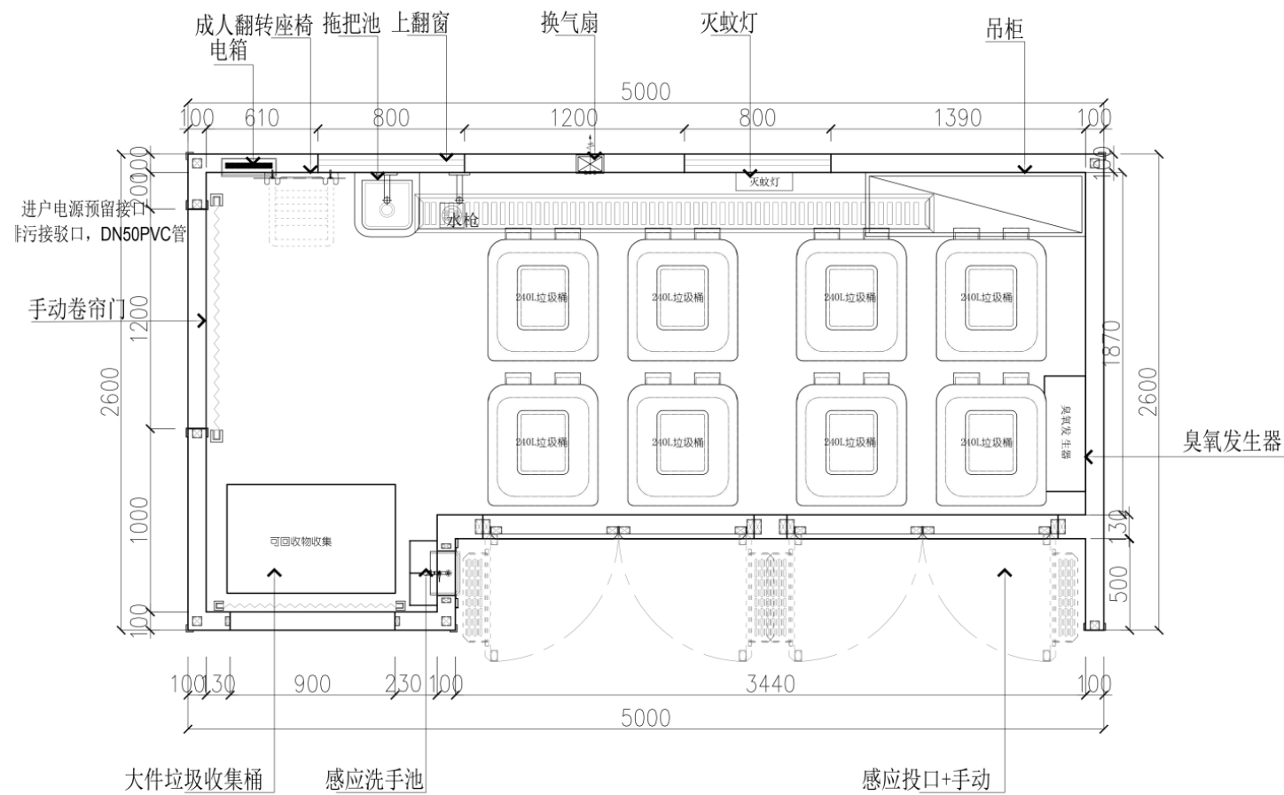
平面布置图
