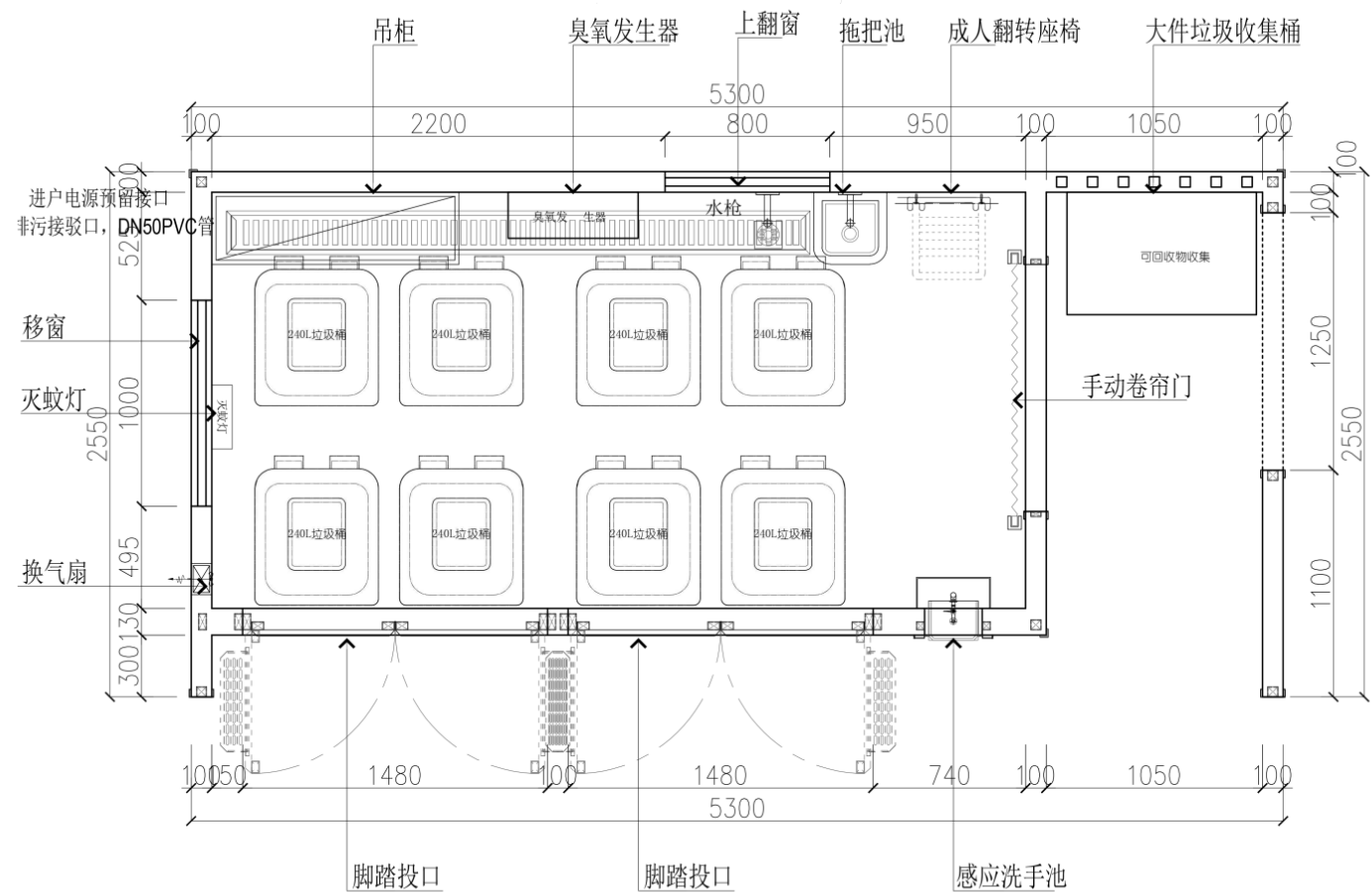
平面布置图
