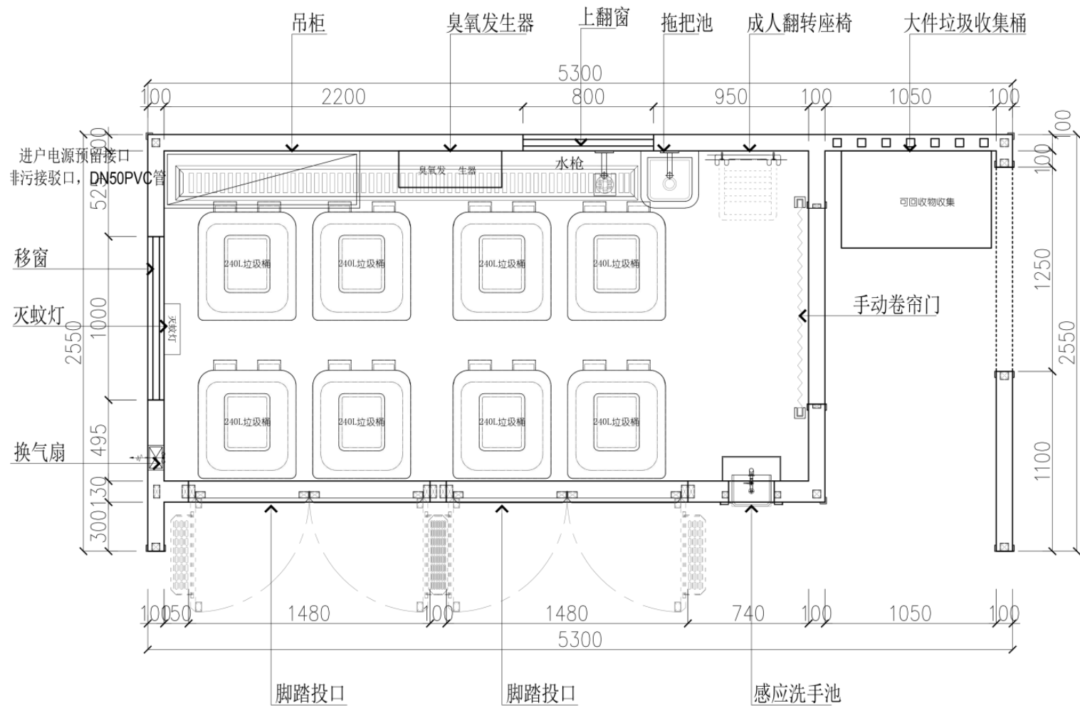
平面布置图
