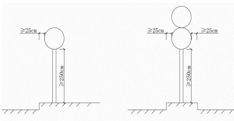
图-1 单柱式
