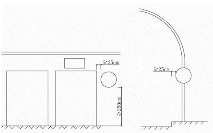
图-3 附着式
