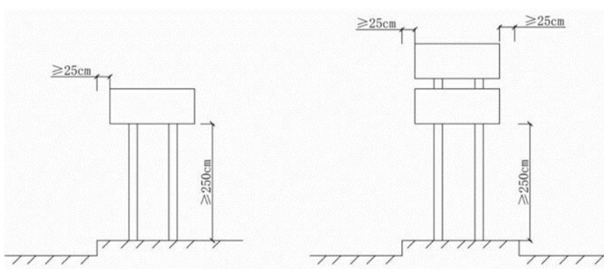
图-2 双柱式
