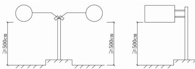
图-4 悬臂式（道路净空高度为 4.5m 时）
