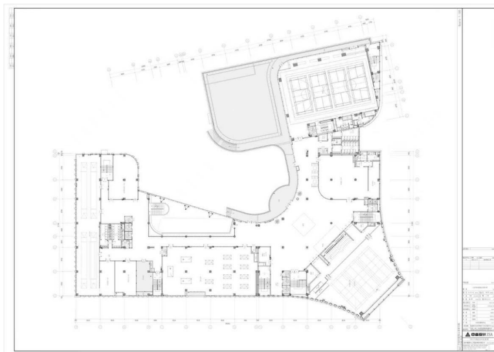
三层平面图
