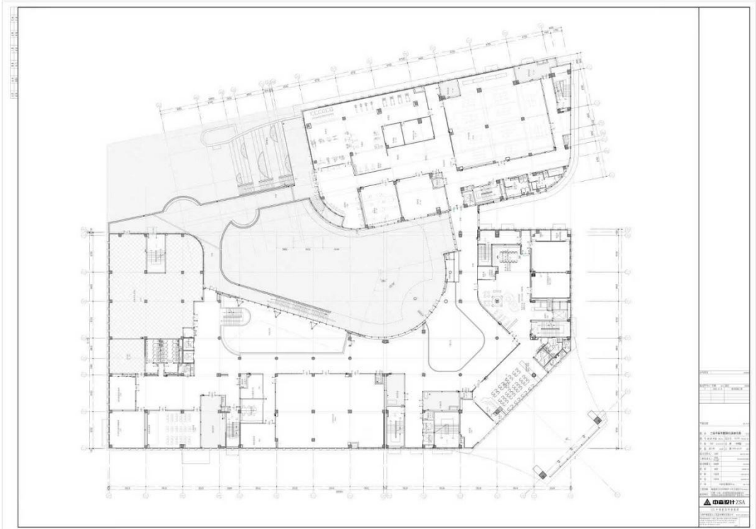
二层平面图
