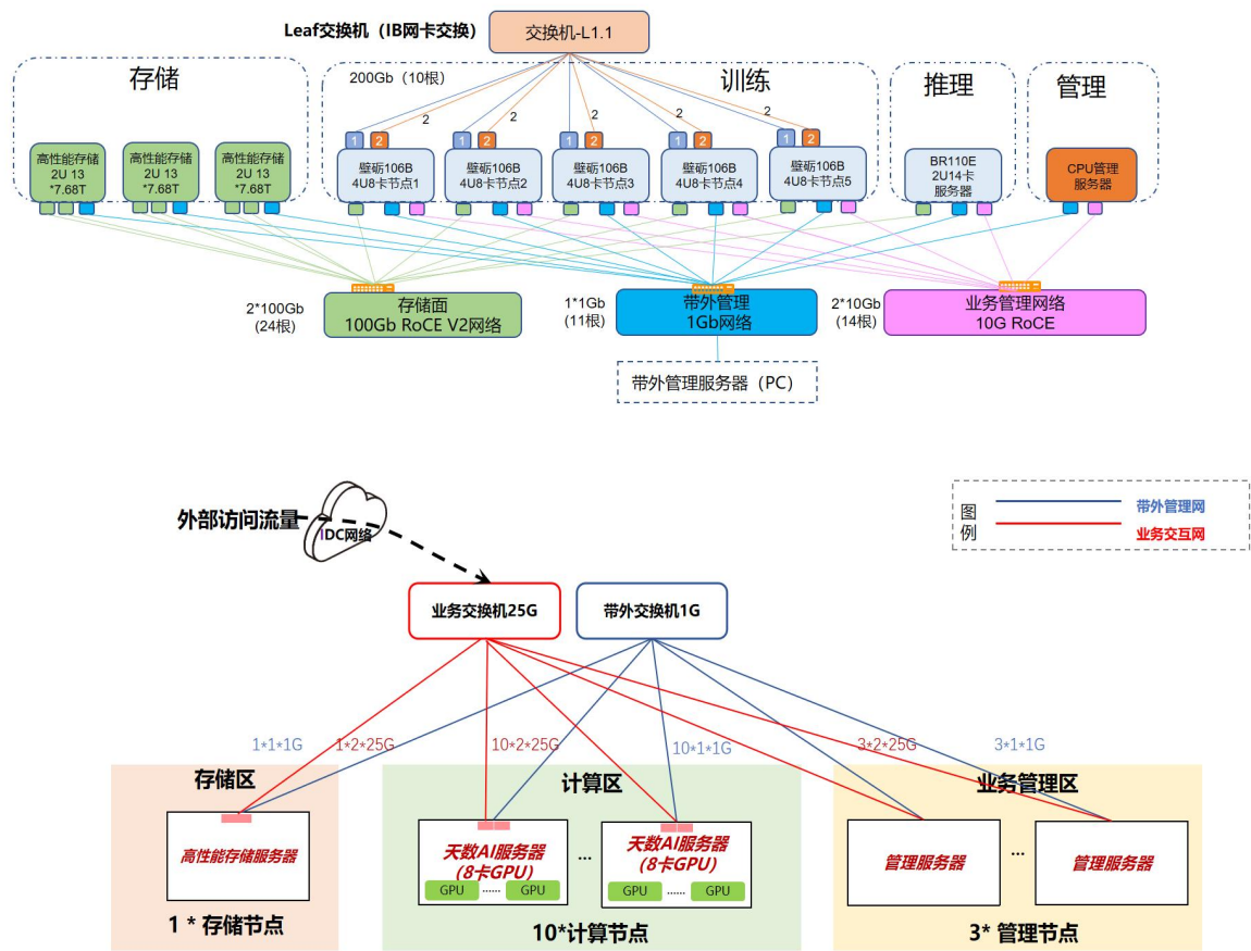
AI参数面-多机通信网络 200Gb IB
