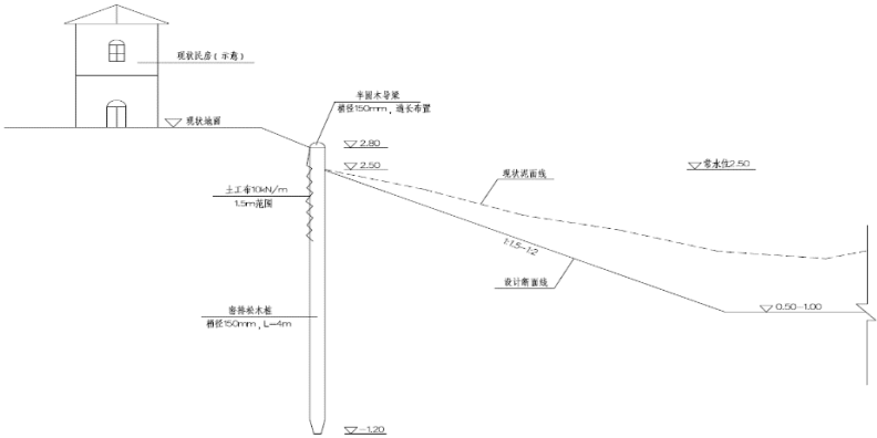
木桩护岸结构图
