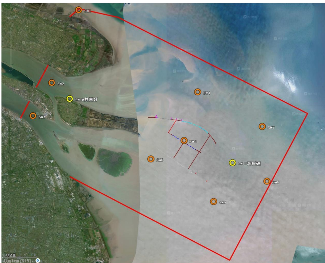
图 4 水文动力监测站位图
