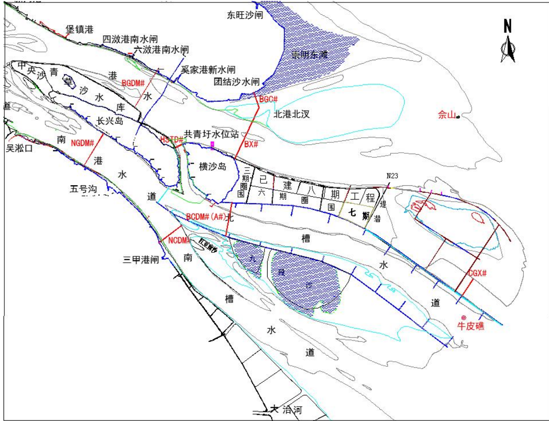
图 3 ADCP 断面监测布置图
