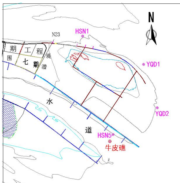
图 2 固定垂线监测布置图
