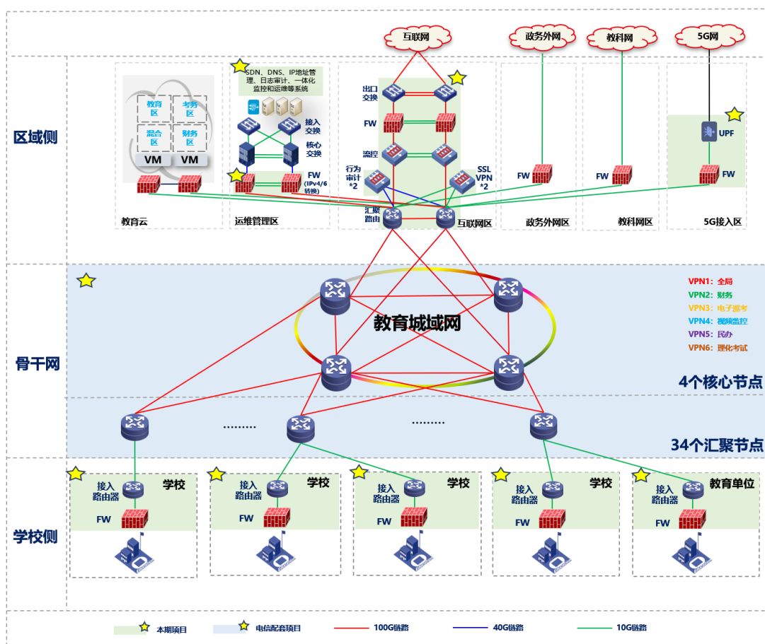
图 1 浦东教育城域网架构拓扑
