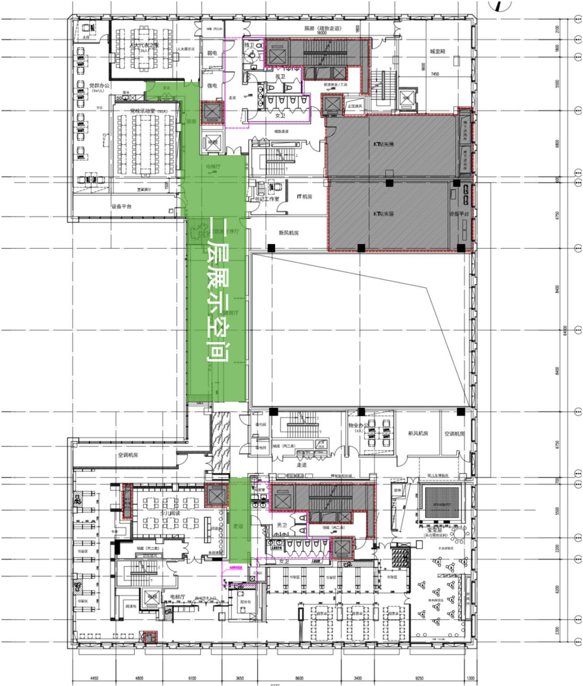
二层平面图（绿色标注部分）
