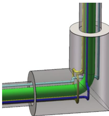
图7 特殊弯头
