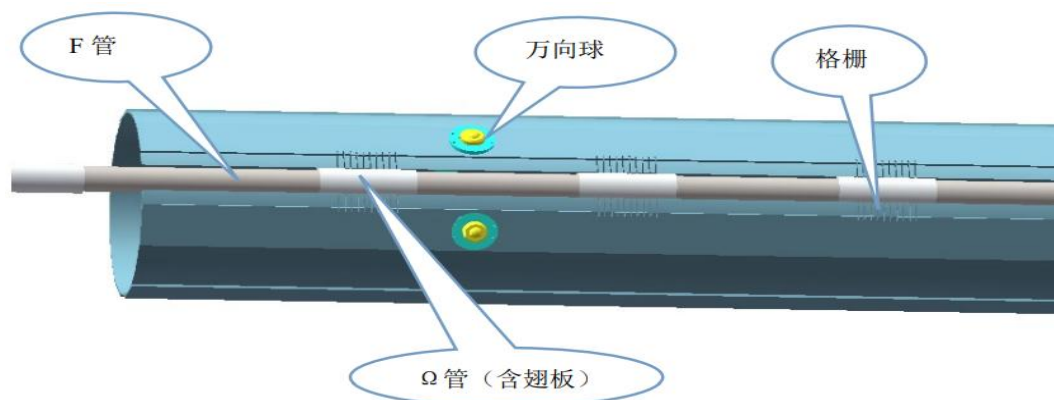
图4 冷屏
