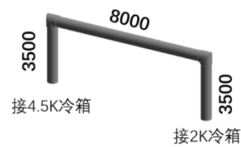
图1 五通道传输线（4.5K冷箱-2K冷箱）
