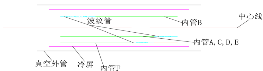
图5 过渡段
