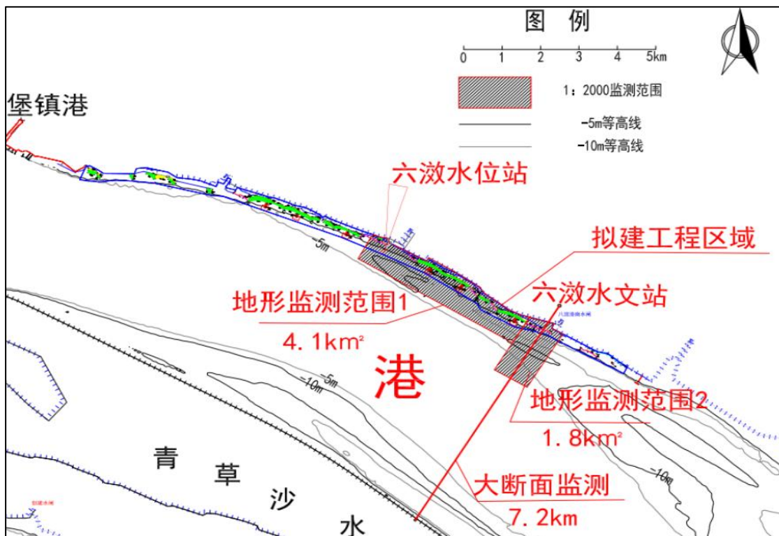
图4 六激港水文站区域监测断面布设示意图（断面不重复布置）
