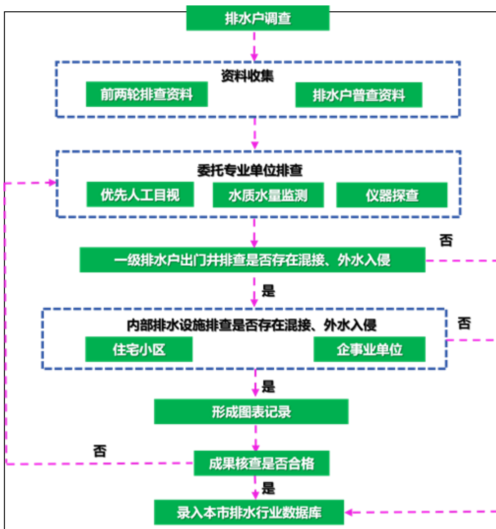
图 3 排水用户出口核查技术路线
