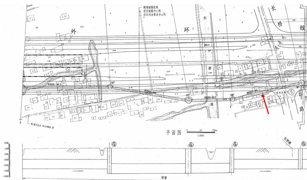
图 1.2.1-1 Φ3000 污水总管竣工资料
