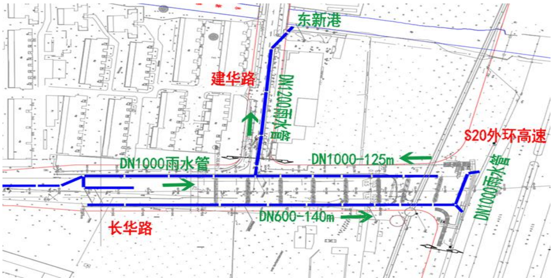
图 1.4-1 长华路（外环路北-外环路南）雨水管道设计图
