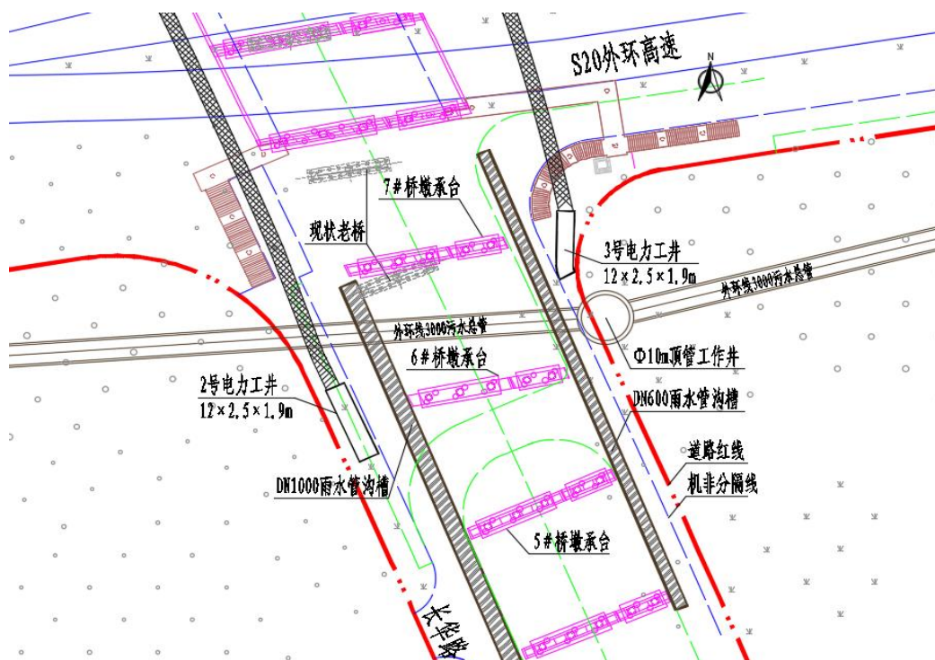
图 1.2.1-2 本工程与Φ3000 污水总管平面位置关系图
