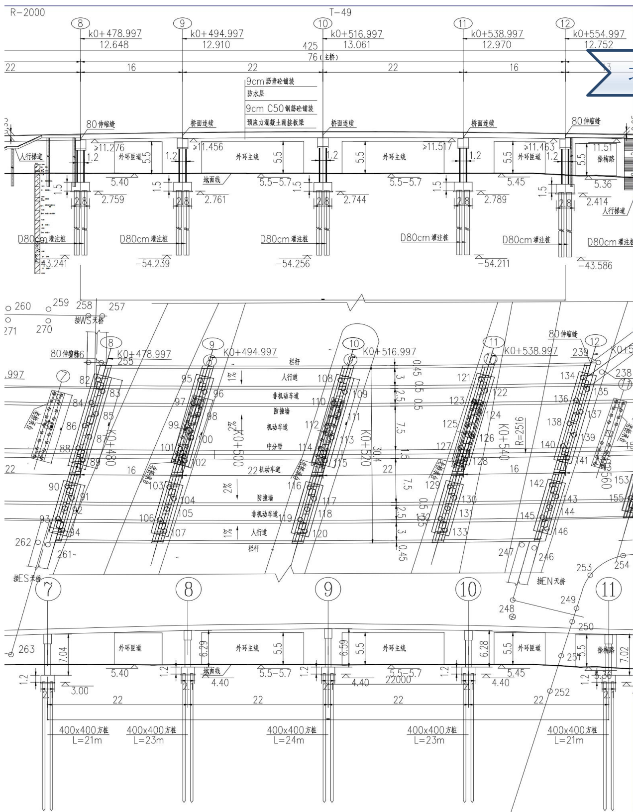
新老桥平、剖面位置关系图
