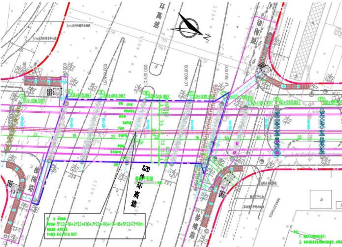
图 1.2-1 拟建桥墩与 S20 关系图
