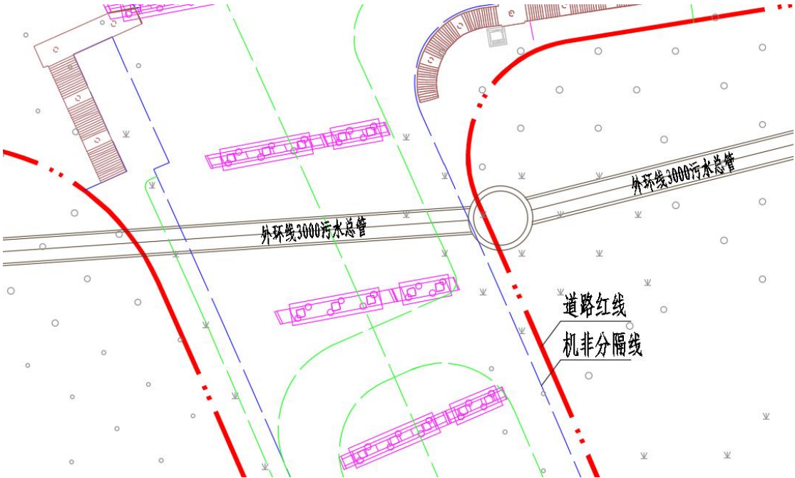
复位道路与Φ3000 污水总管平面位置关系
