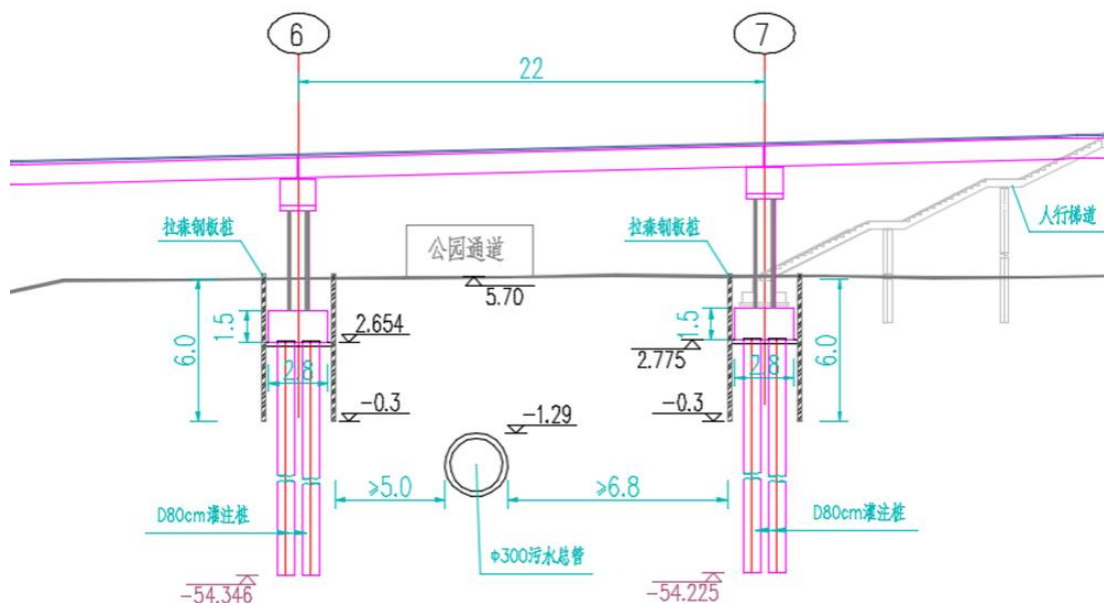
桥梁基础与污水总管立面位置关系图
