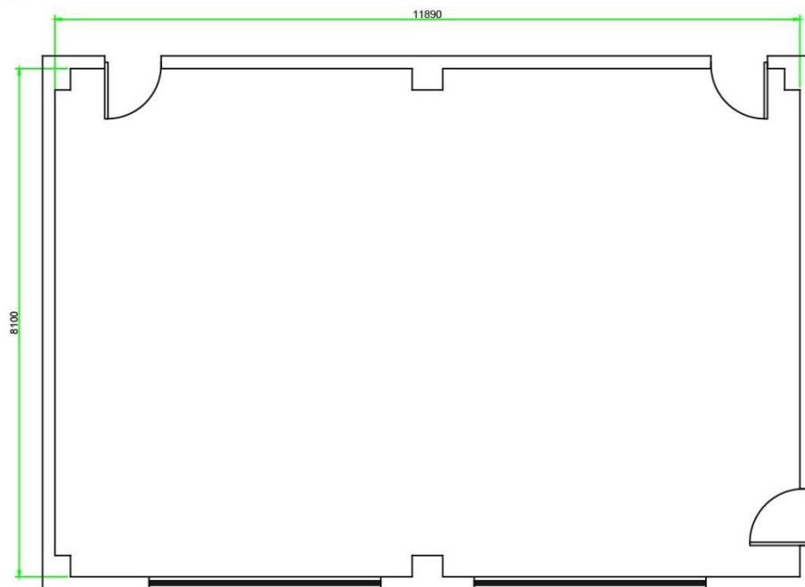
化学实验室平面图(56人)
