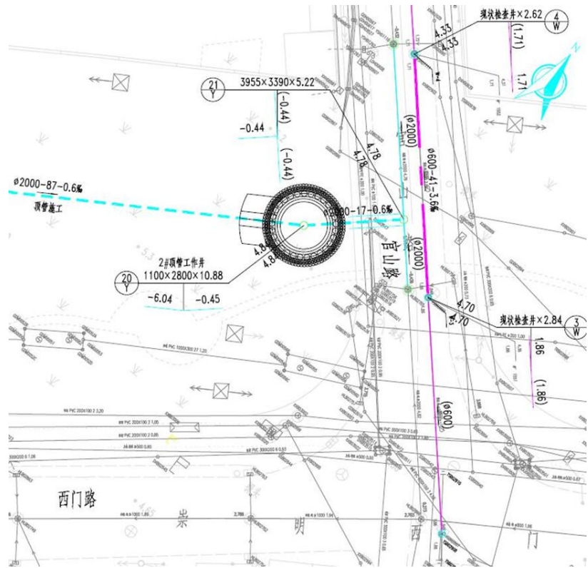
图 1.1.5 2#顶管工作井
