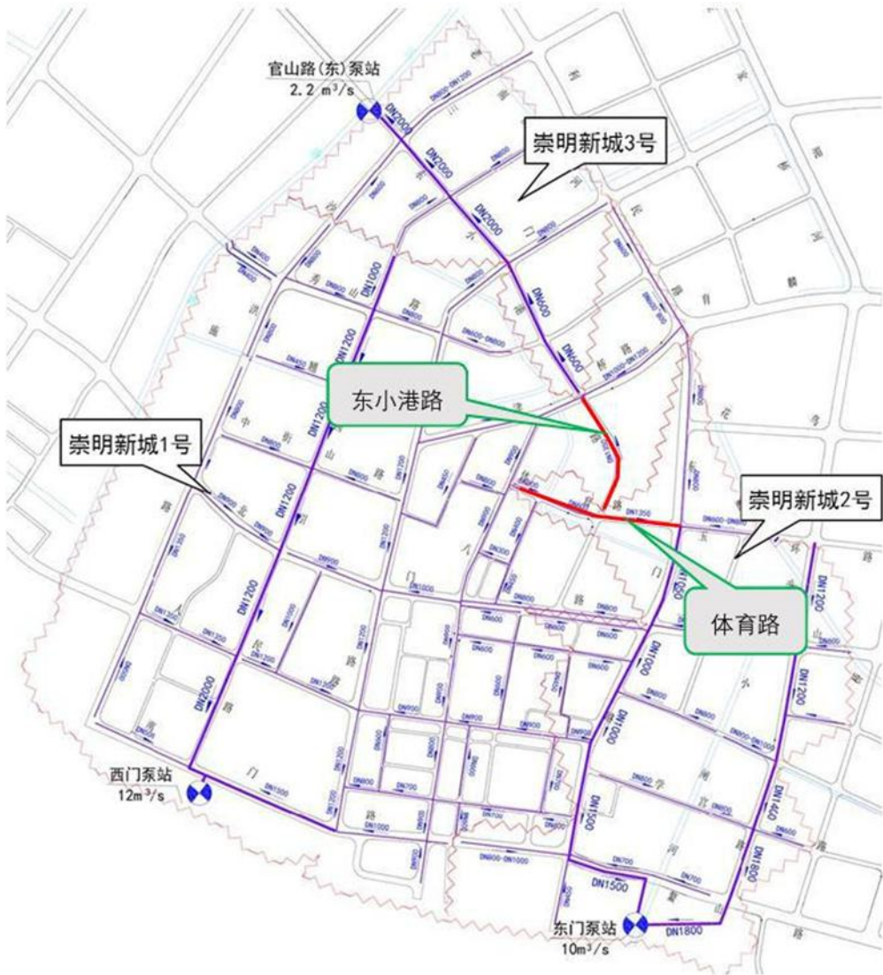
图 1.1.1 设计概况
