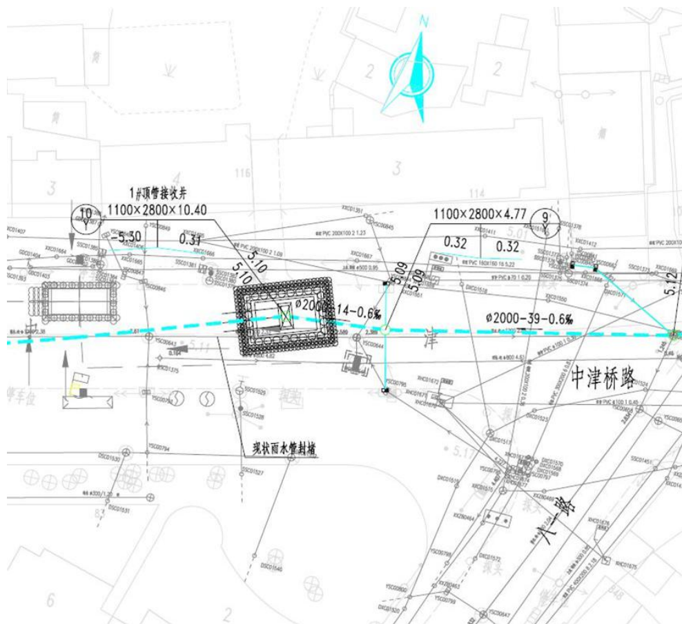
图 1.1.2 1#顶管接收井
