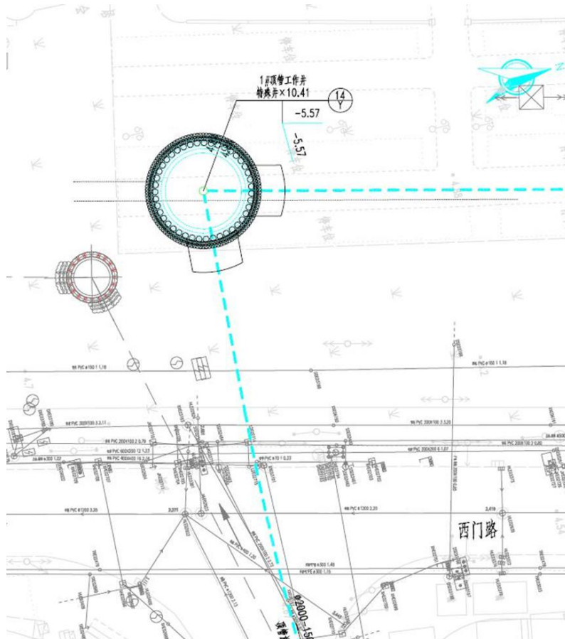
图 1.1.3 1#顶管工作井
