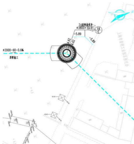
图 1.1.4 2#顶管接收井
