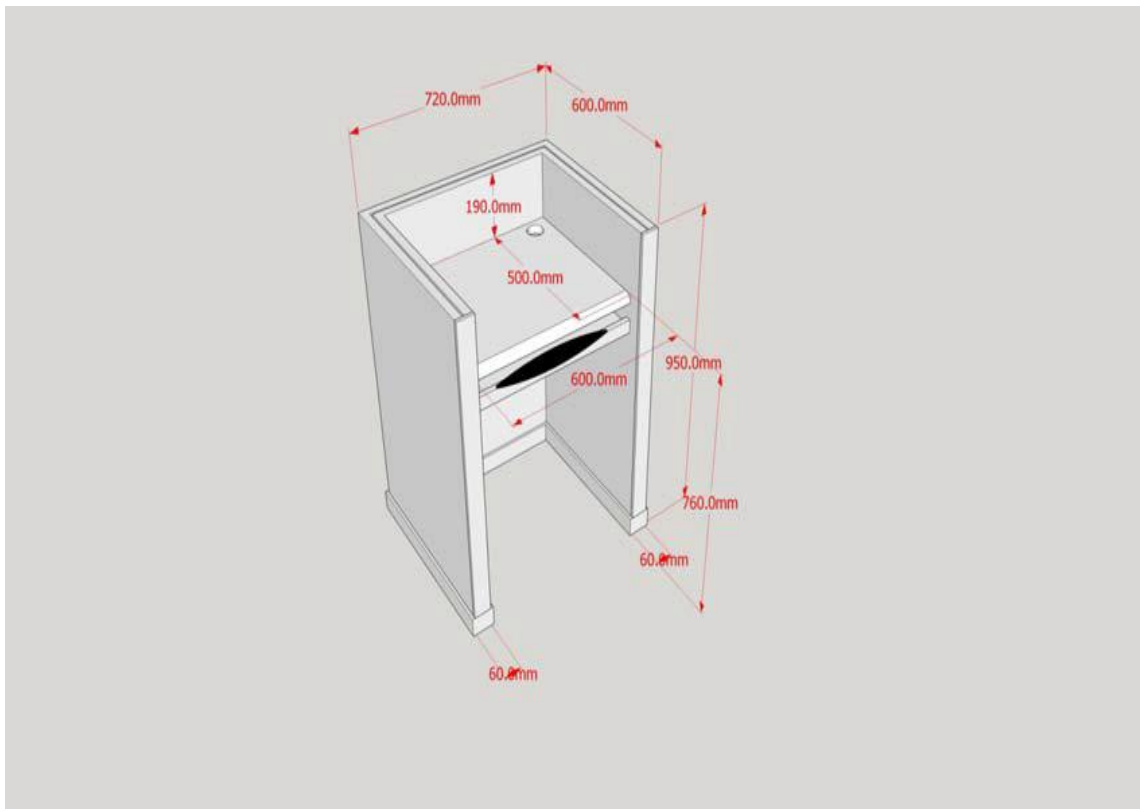
单人升降卡座（非标）降下时尺寸图
