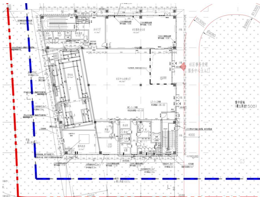
1 号楼第一层平面图
