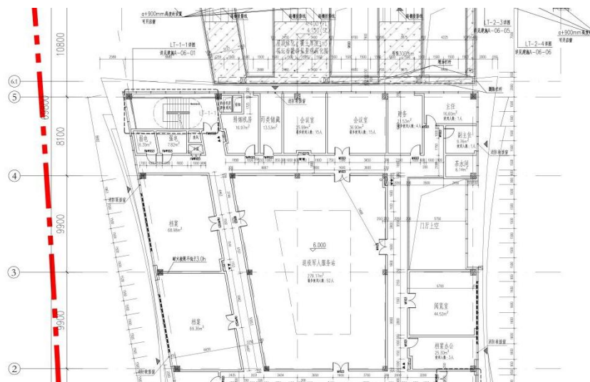
1 号楼第二层平面图
