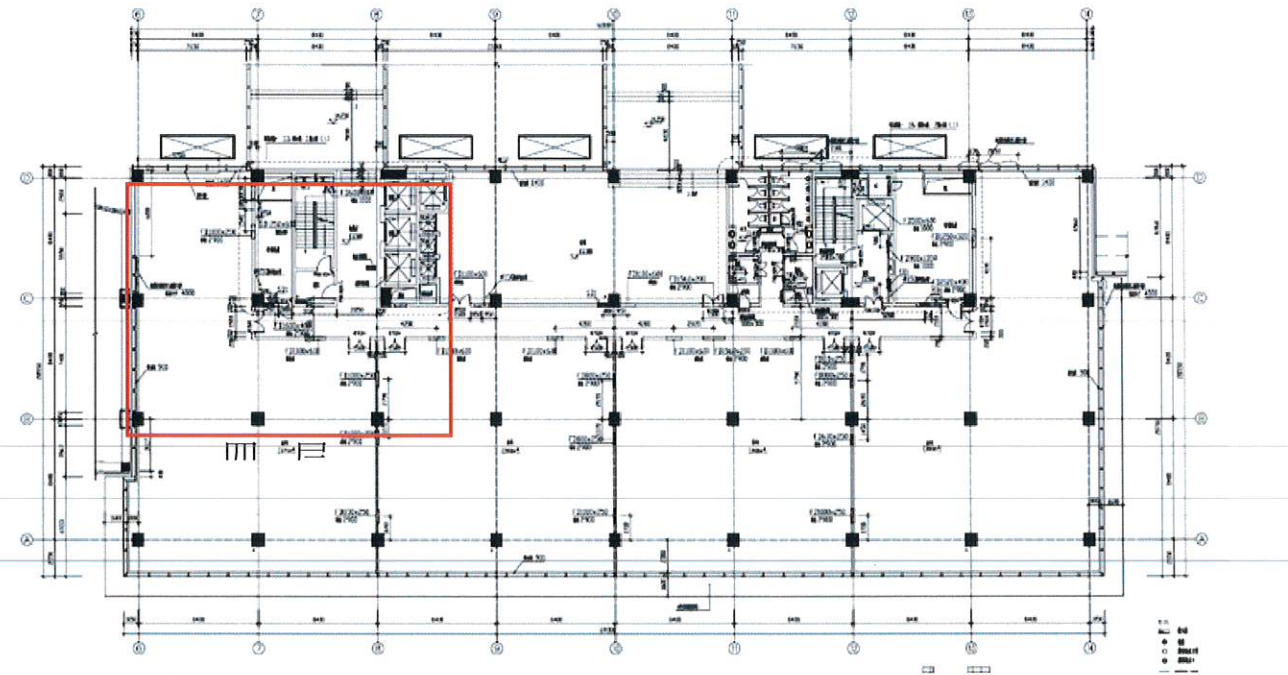
四层平面图
