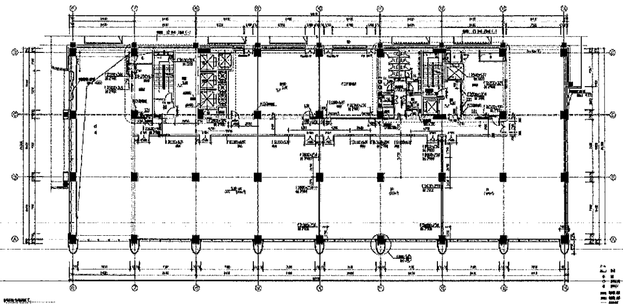
二层平面图
