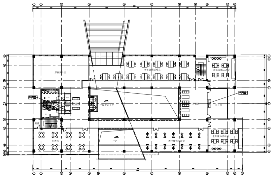
三层平面图
