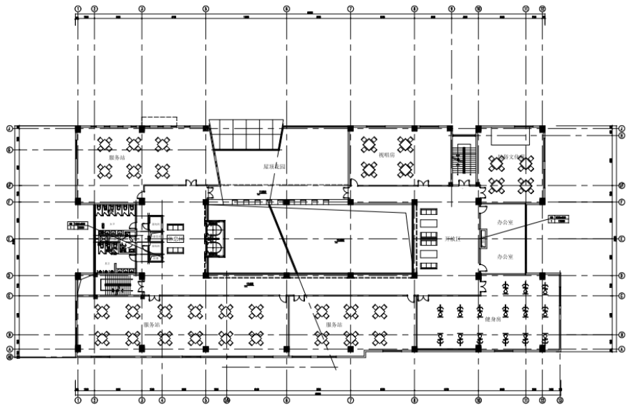
四层平面图
