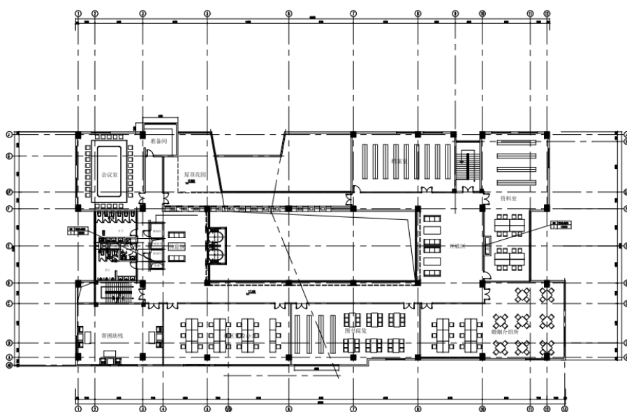
五层平面图
