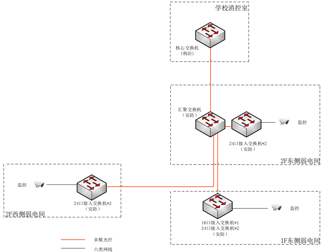
设备网络拓扑图:
