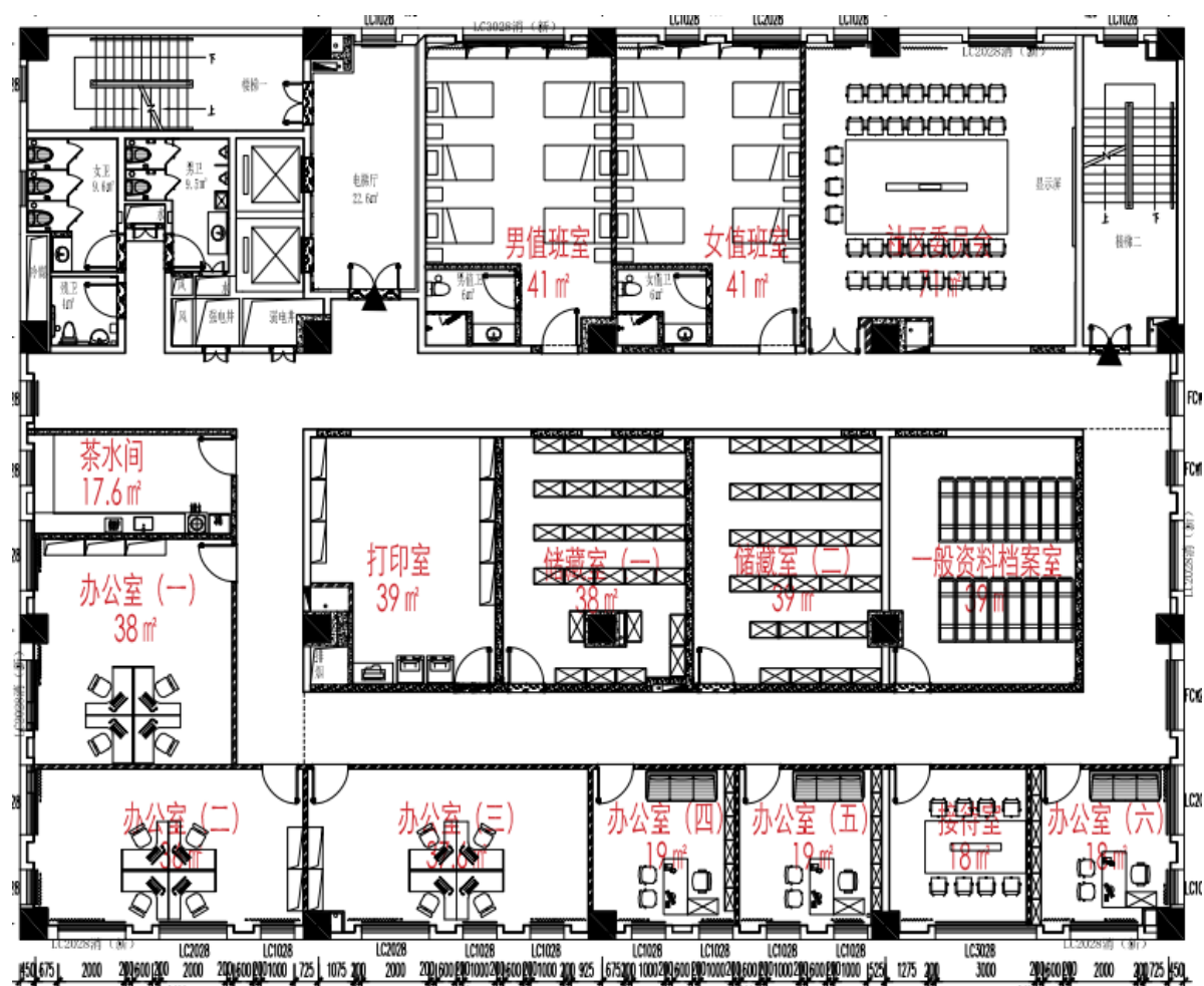
A 区塔楼五层平面图
