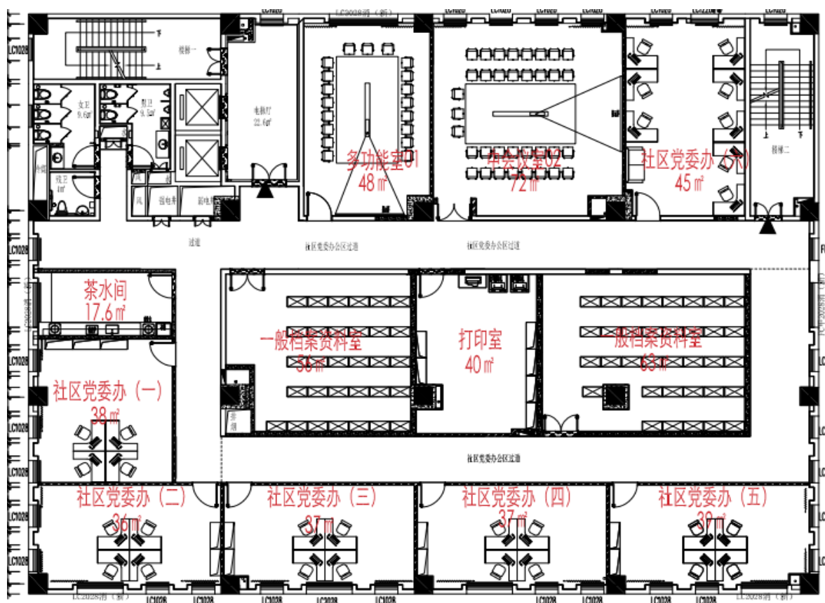
A 区塔楼四层平面图
