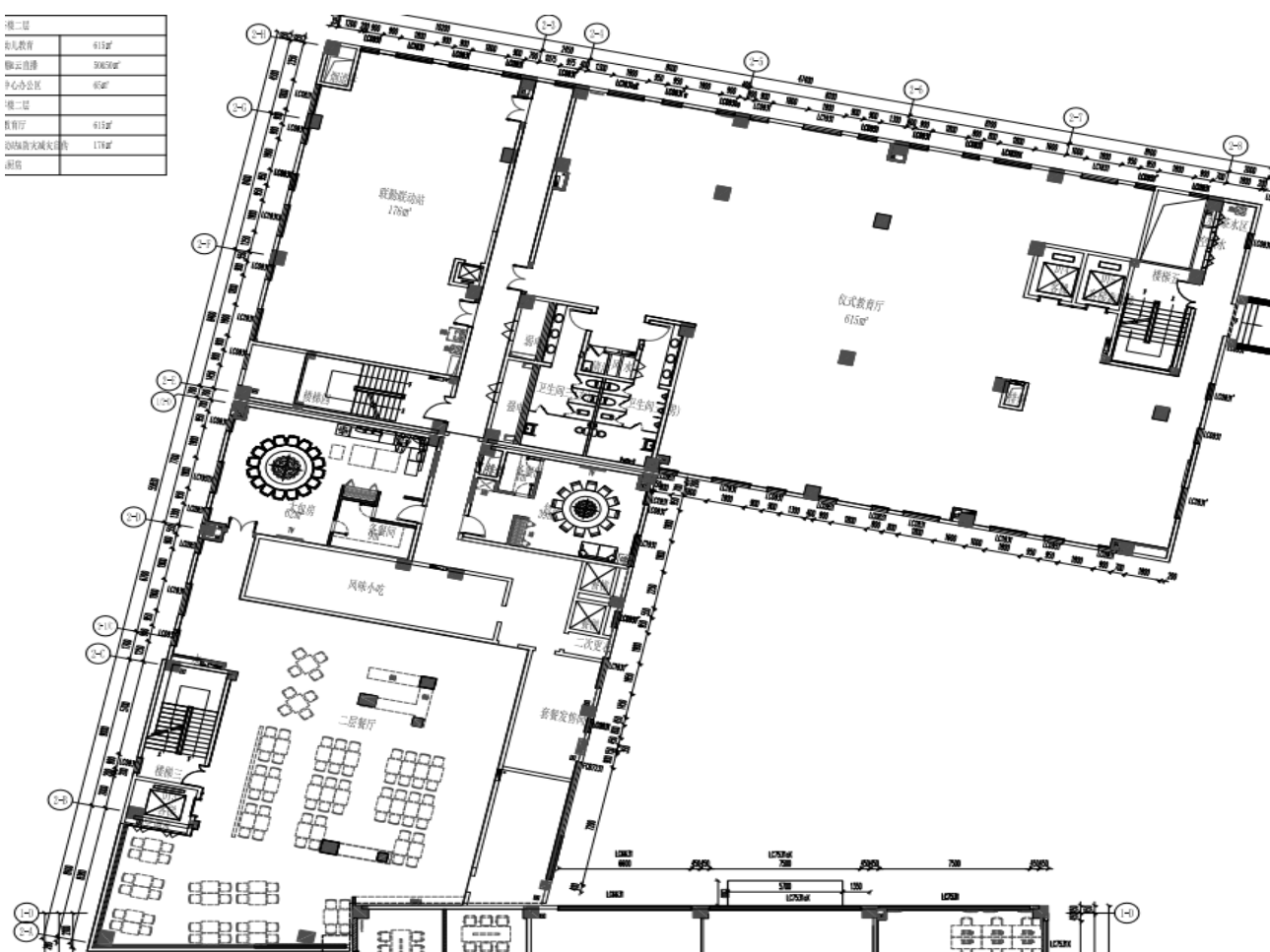
B 区裙楼三层平面图
