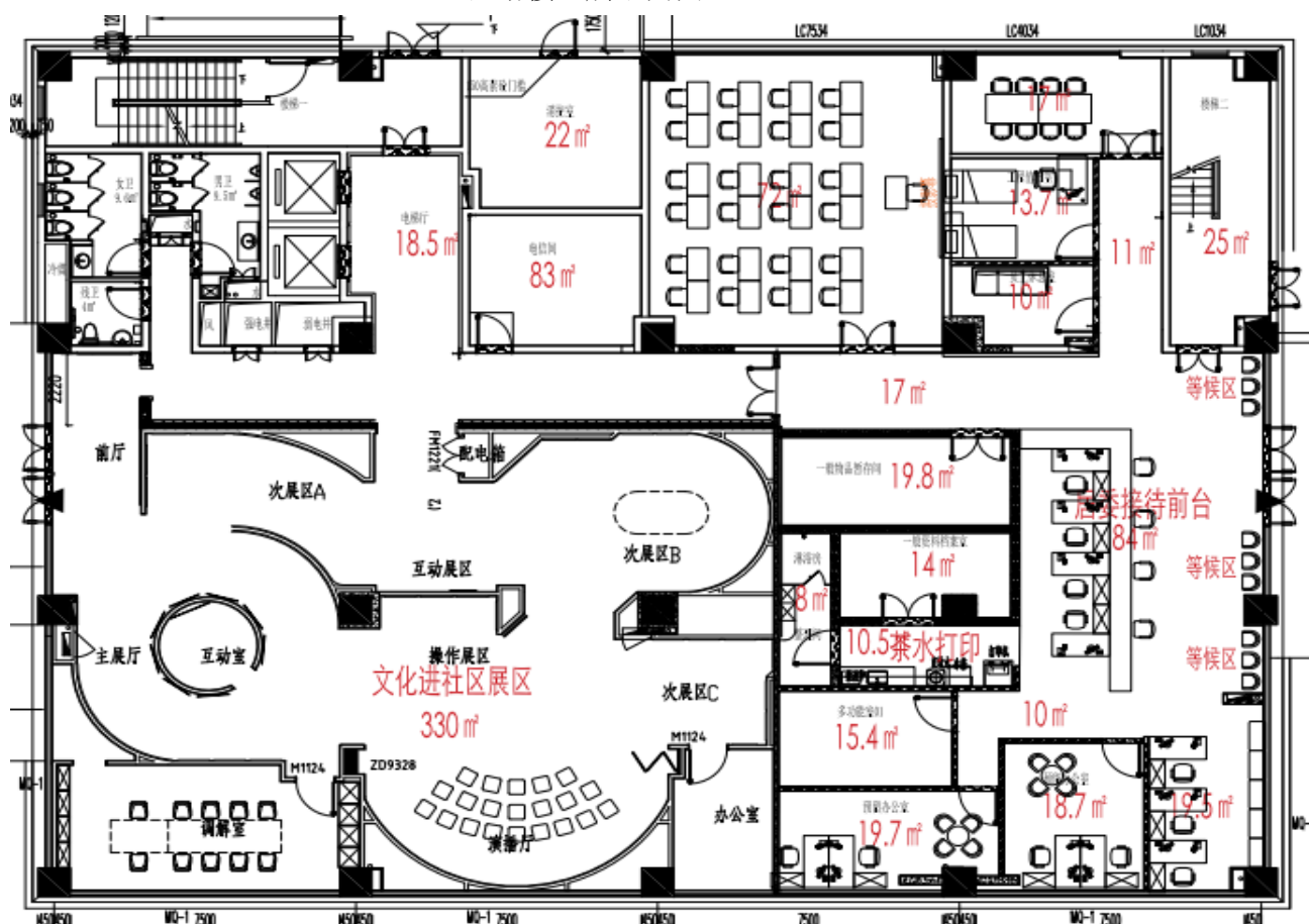
A 区塔楼一层平面图
