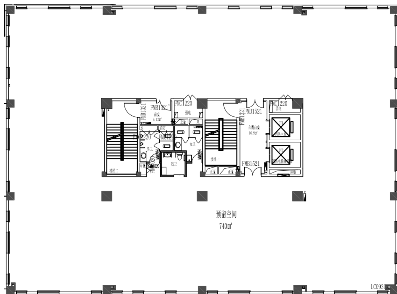
B 区塔楼八层平面图
