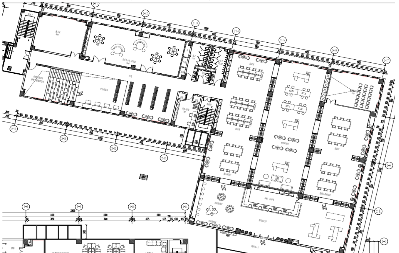
A 区裙楼二层平面图
