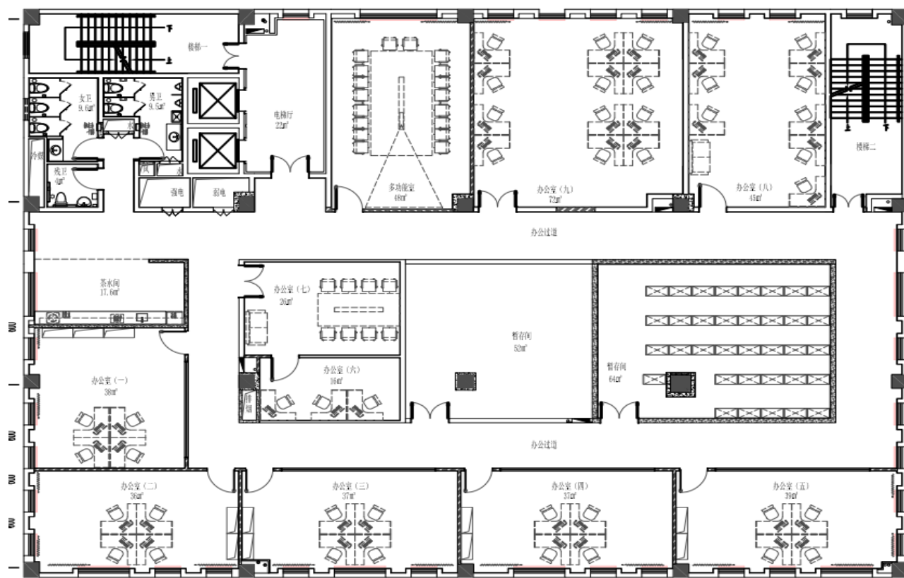
A 区塔楼八层平面图
