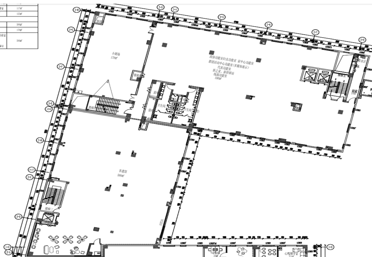
B 区裙楼四层平面图
