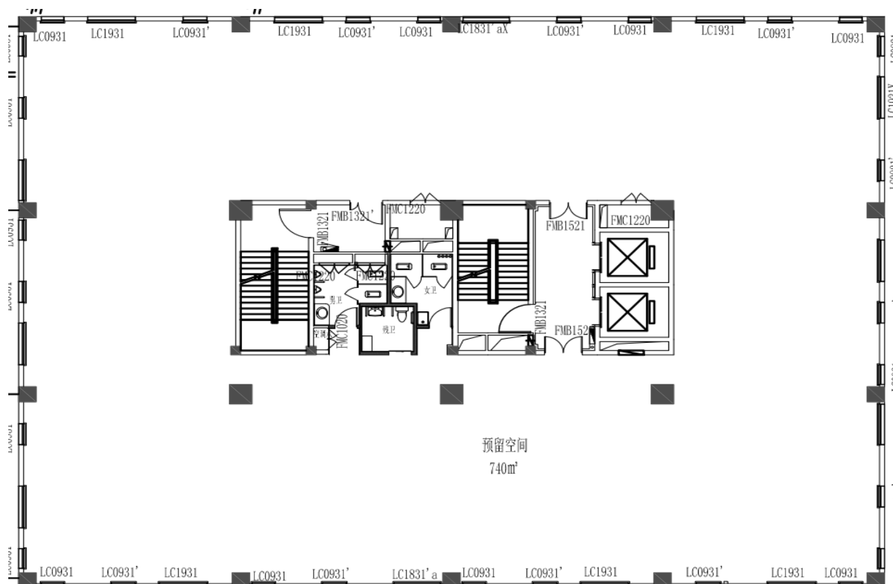
B 区塔楼八层平面图
