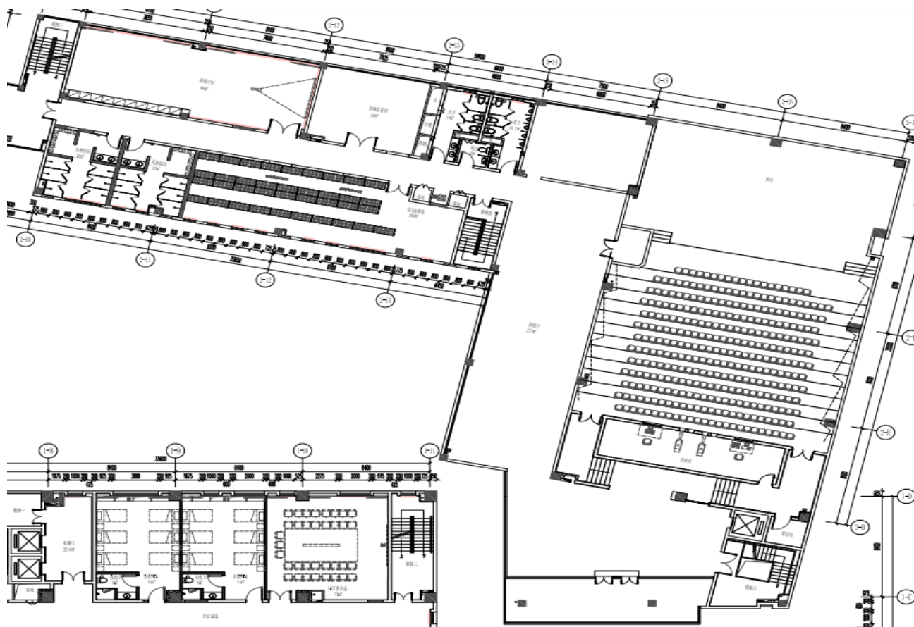
A 区裙楼五层平面图
