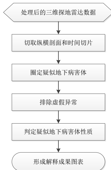
图 3.7.1 三维探地雷达资料解译流程图
