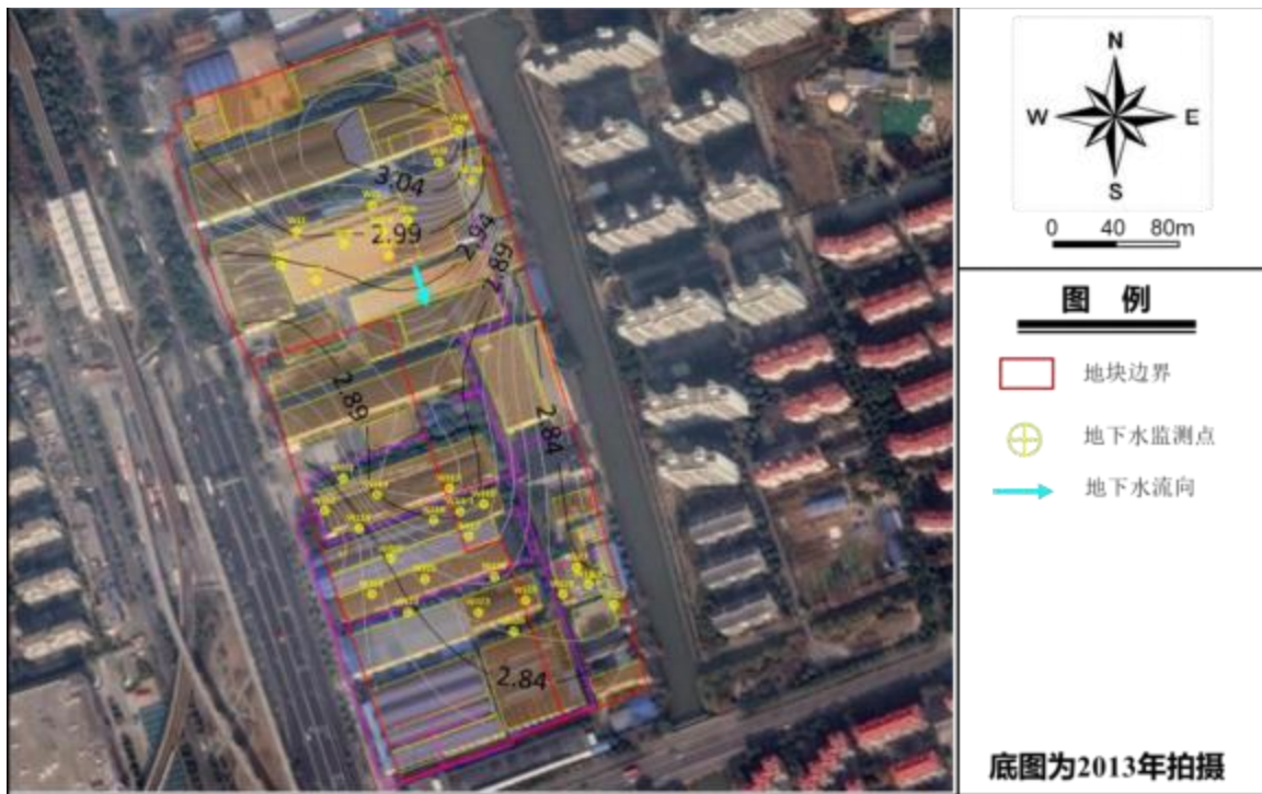
图2.3-3 地下水流向图
