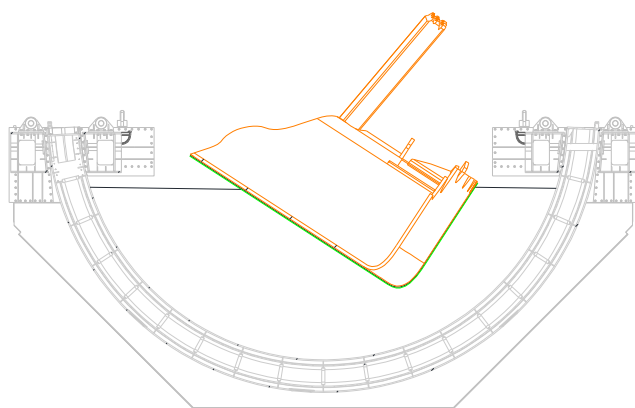
船体在沉箱中横剖面
