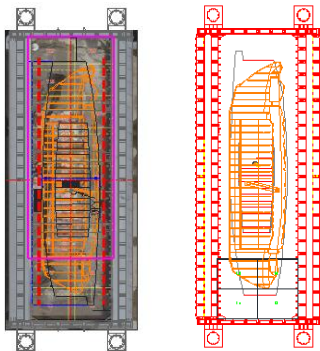
开挖范围示意图（粉红框标识区域）
